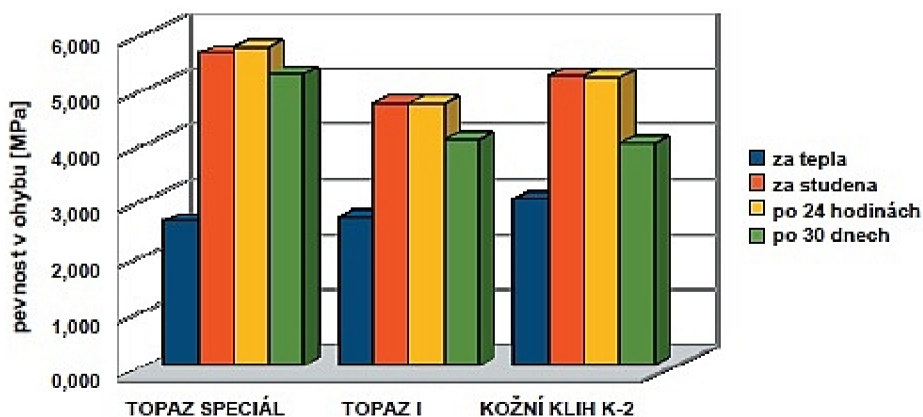
Obr. 16 Pevnosti zkušebních trámečků s pojivý na bázi klišů [23].
