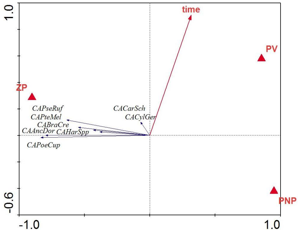
Obrázek 5: RDA model ukazující distribuci pro jednotlivé druhy střevlíků v závislosti na odchytných metodách Pozn. CAAncDor – Anchomenus dorsalis , CABraCre – Brachinus crepitans , CACarSch – Carabus scheidleri , CACylGer – Cylindera germanica , CAHarSpp – Harpalus spp. , CAPoeCup – Poecilus cupreus , CAPseRuf – Pseudoophonus rufipes , CAPteMel – Pterostichus melanarius
