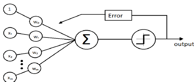
Graf 2: Schéma perceptronu
