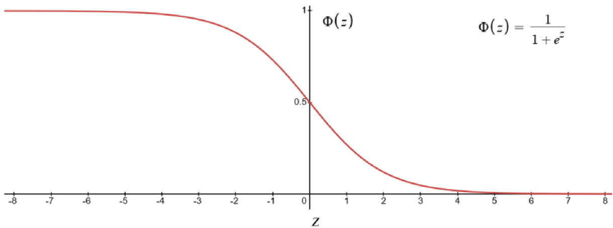
Graf 3: Sigmoida
