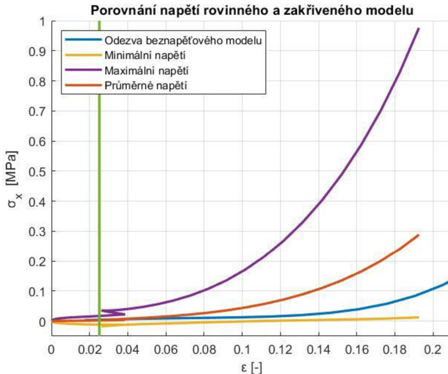
Obr. 6.11 Porovnání odezvy skutečného napětí-přetvoření rovinného (beznapětového) a rozvinutého modelu. Zeleně odděleno rozvinutí a natahování zakřiveného modelu
