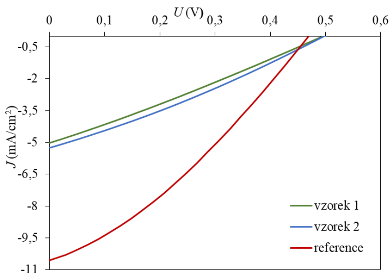
Obr 21. V-A charakteristika referenčního a finálních vzorků (aktivní plocha 1 cm 2 )
