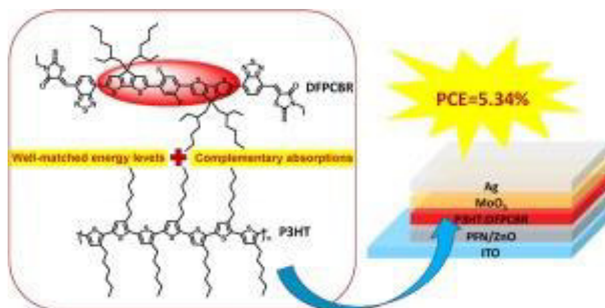
Obr 8. OSC s aktivní vrstvou P3HT a DFPCBR (OSC bez fullerenu) [12]
