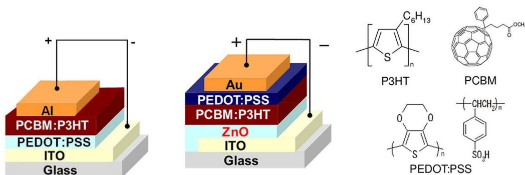
Obr 12. Klasická a invertovaná struktura OSC
