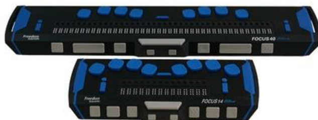
Obrázek 14- Braillový zobrazovač ( https://www.galop.cz/katalog_detail.php?produkt=45 )
