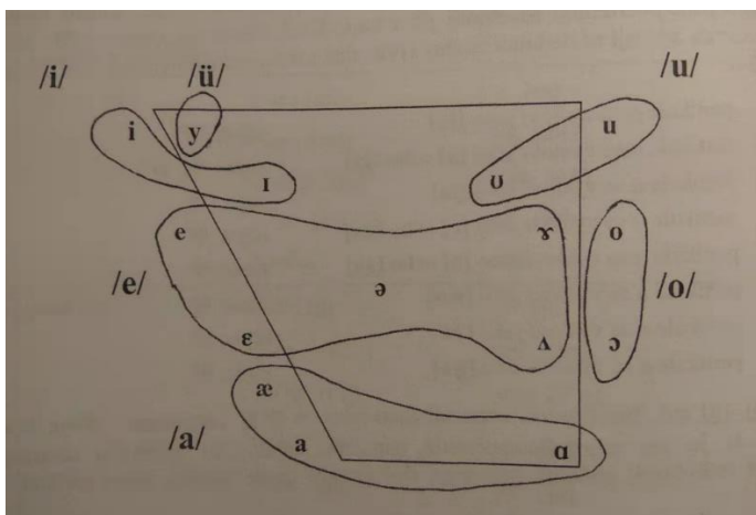
Obrázek 2 Vokalický čtyřhelník
