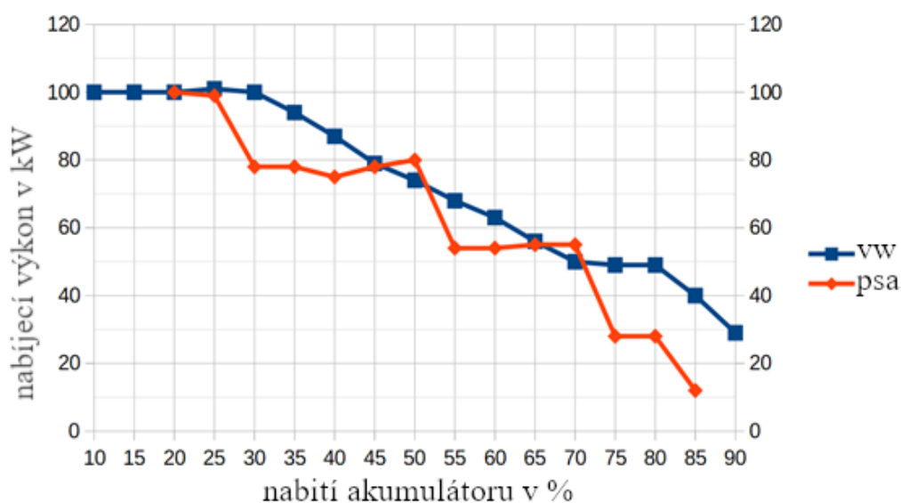
Obrázek 2 Nabíjecí křivka [4]
