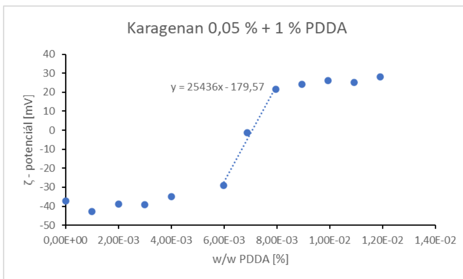
Graf č. 8: Závislost zeta potenciálu stabilizovaných koloidních částic stříbra 0,05 % \kappa - Karagenanem na koncentraci PDDA
