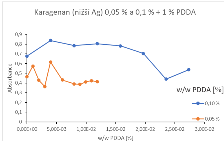
Graf č. 12: Závislost absorbance při vlnové délce 396 nm stabilizovaných koloidních částic stříbra 0,05 % a 0,1 % κ-Karagenanem na koncentraci 1 % (w/w) PDDA
