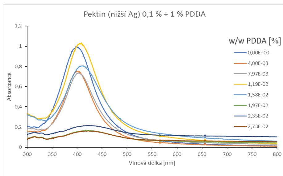
Graf č. 15: Absorpční spektrum stabilizované koloidní disperze stříbra 0,1 % pektinem při destabilizaci 1 % (w/w) PDDA
