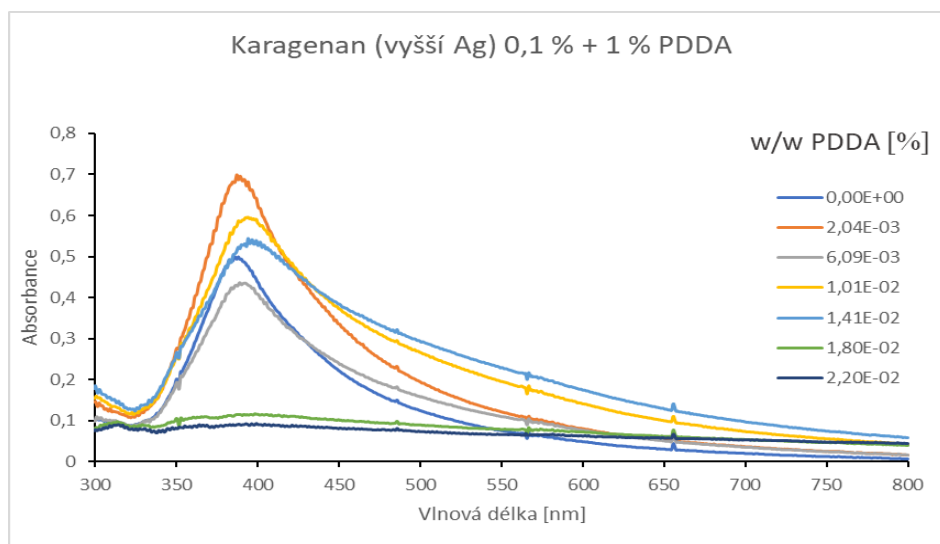
Graf č. 25: Absorpční spektrum stabilizované koloidní disperze stříbra 0,1 % κ-Karagenanem při destabilizaci 1 % (w/w) PDDA
