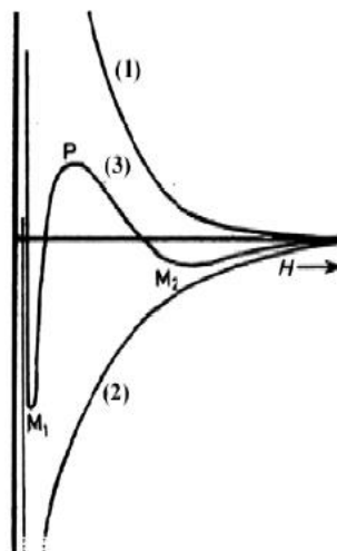
Obrázek č. 3: Křivka integrační energie (3) v závislosti na rostoucí vzdálenosti H , (1) křivka odpuzivých sil (2) křivka přitažlivých sil [3]
