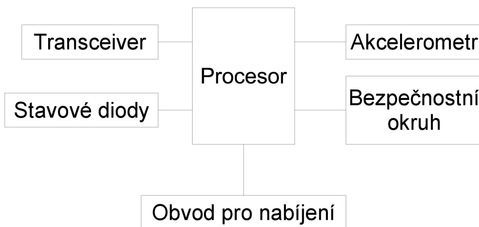
Obrázek 2.2: Měřicí modul - blokové schéma
