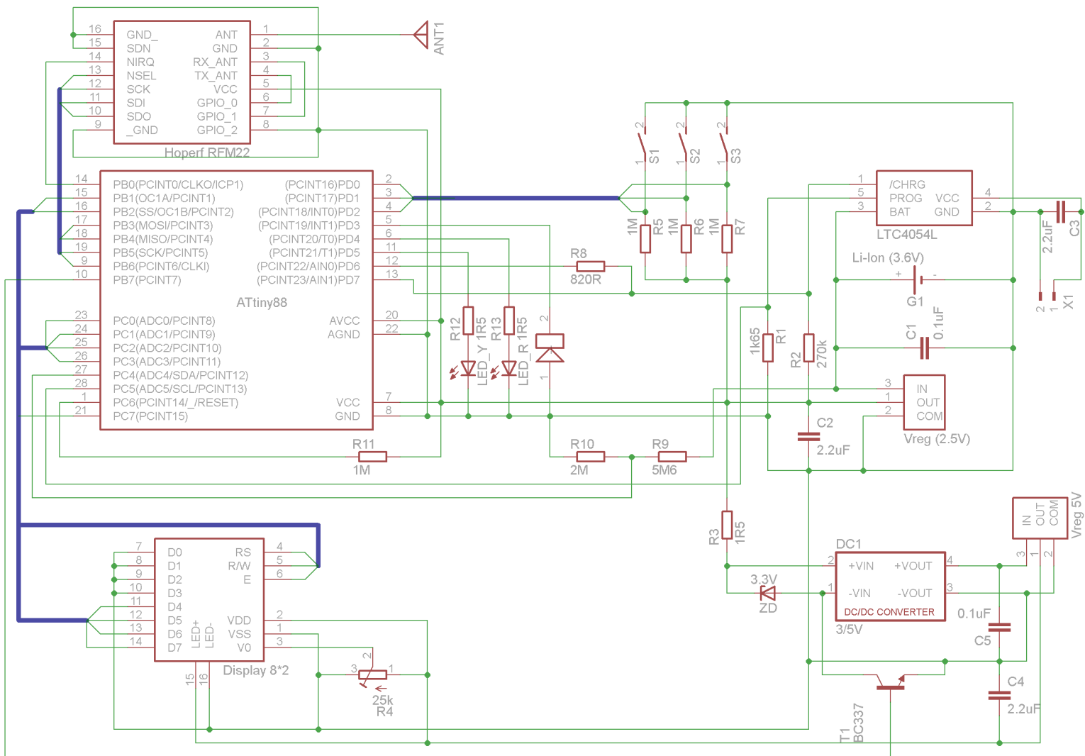
Obrázek 2.20: Řídící modul – schéma zapojení
