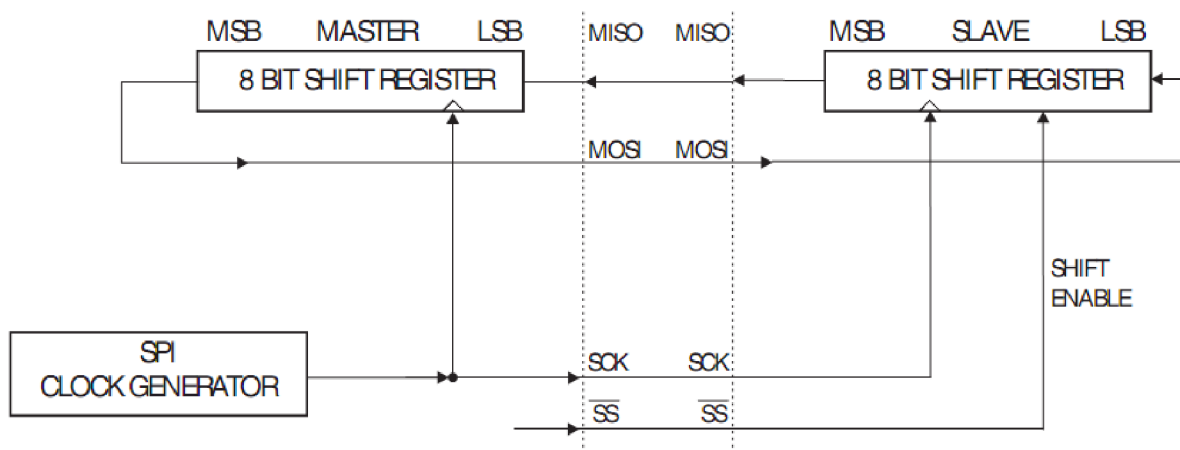
Obrázek 2.3: Komunikace pomocí rozhraní SPI
