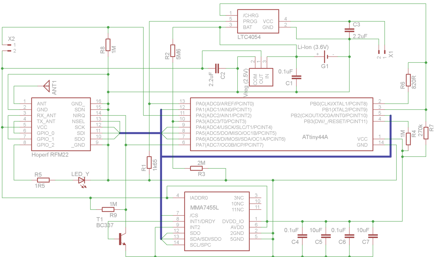
Obrázek 2.21: Měřičí modul - schéma zapojení
