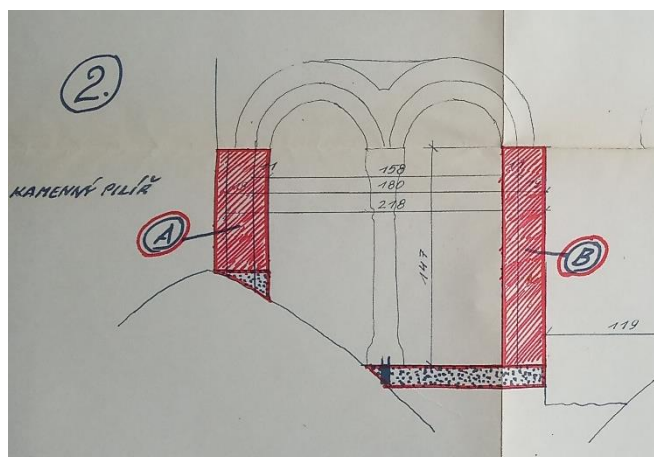
Obr. VIII Aleš Rozehnal, Plán rekonstrukce okna č. 1 (ořezáno), 1980, perokresba, Pozůstalost AR, archiv MUO, složka č. 87. Písmeny A a B jsou značeny pilíře z bílých cihel.
