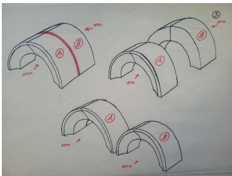
Obr. 26 Aleš Rozehnal, Rozříznutí okenního záklenku kvůli rekonstrukci okna č. 2, 1980–1985, perokresba, Pozůstalost AR, archiv MUO, složka č. 305.
