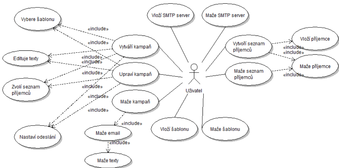
Obrázek 8 : Use case diagram uživatelských funkcí (zdroj vlastní)
