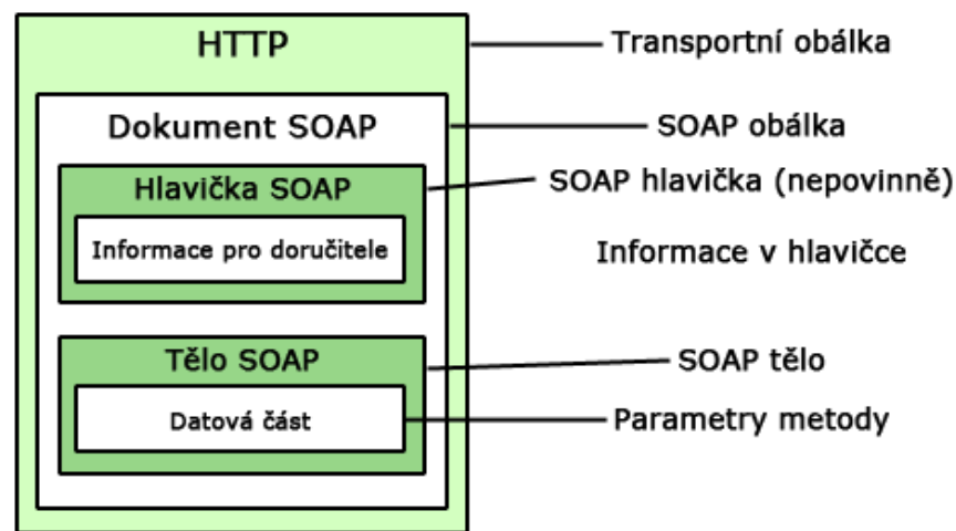
Obrázek 2: Struktura SOAP (zdroj vytvořeno dle [17])
