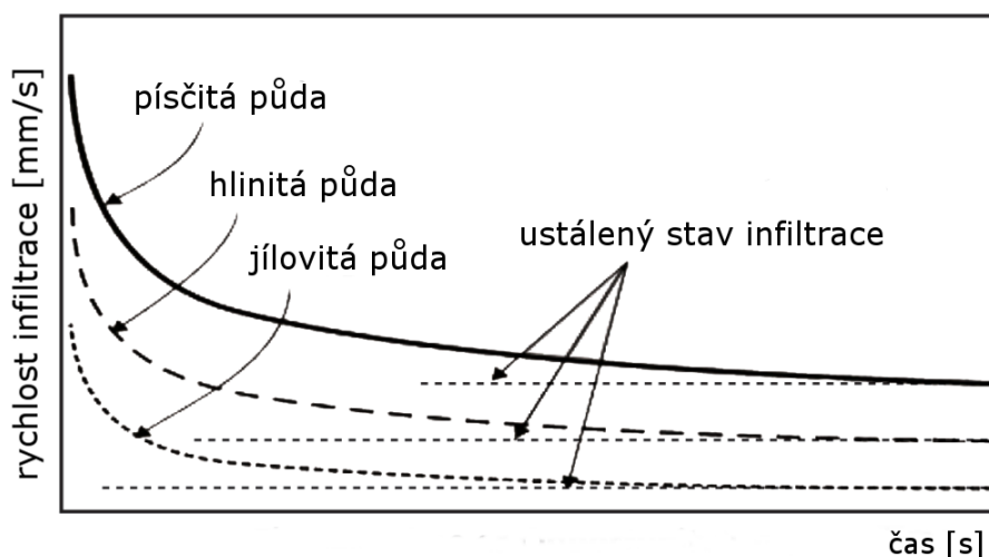
Obrázek 3. Příklad infiltračních křivek pro různé druhy půd (MILLER, 1994) (upraveno: Bárta)
