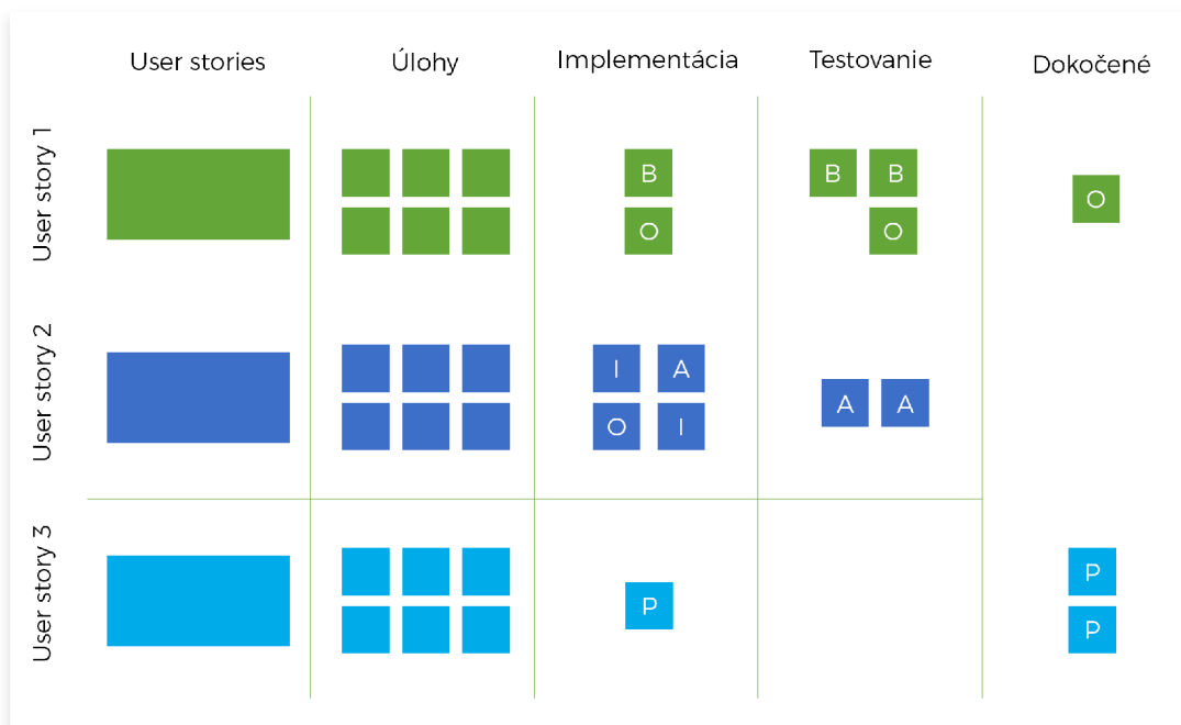
Obr. 3.1: Scrum tabuľa
