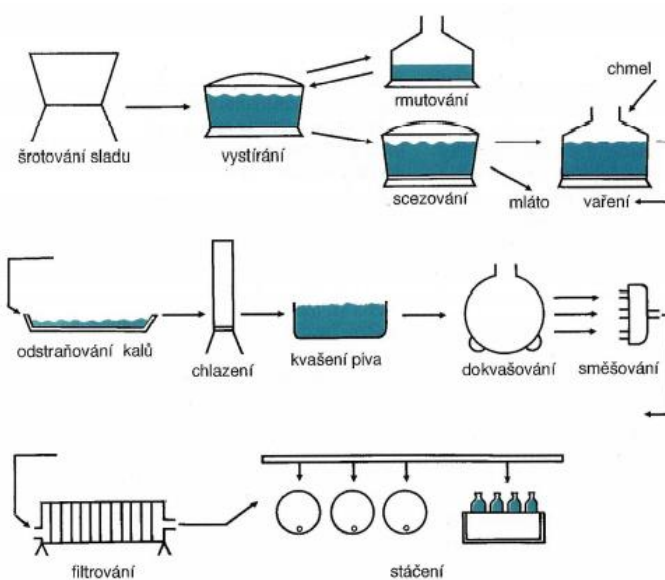
Obrázek 6: Schéma výroby piva (Salač, 2001)
