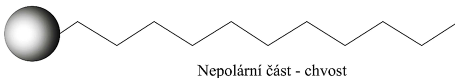
Obr. 15 Schématické znázornění molekuly tenzidu.
