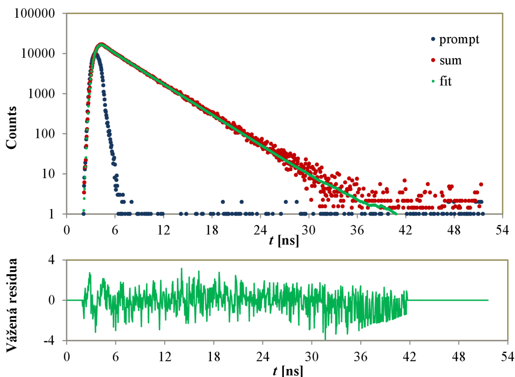
Obr. 20 Příklad vyhodnocení „sumy“ naměřených poklesů fluorescence vzorku s rhodaminem 6G ve směsi glycerol/voda s 86,7% hm glycerolu. Prompt – odezva lampy, sum – suma jednotlivých poklesů fluorescence (při VV a VH orientaci polarizátorů) a fit – proložená funkce. Hodnota \chi_R^2 = 1,103 .
