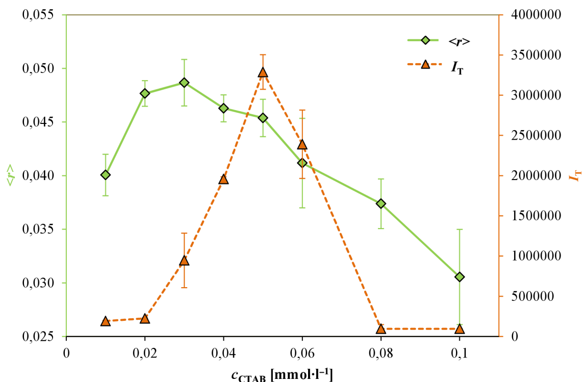
Obr. 28 Závislost totální intenzity fluorescence a anizotropie fluorescence na koncentraci CTAB ve vzorcích obsahující 0,015 g·l -1 Hya ve vodném prostředí.
