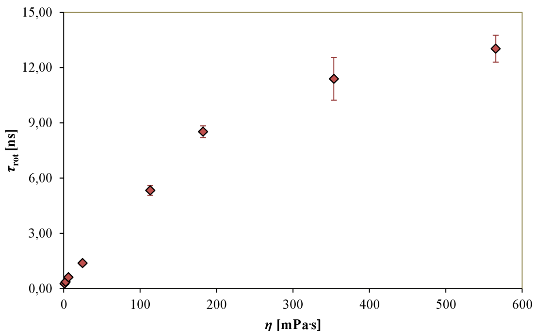
Obr. 25 Závislost rotační korelační doby rhodaminu 6G na viskozitě homogenního prostředí (směs glycerol/voda).
