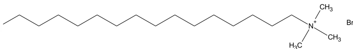
Obr. 18 Molekula CTAB.
