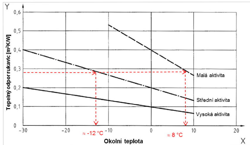
Obrázek 8.5: Graf pro určení použitelnosti vzorku č. 4
