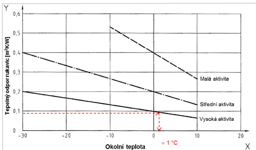
Obrázek 8.2: Graf pro určení použitelnosti vzorku č. 1
