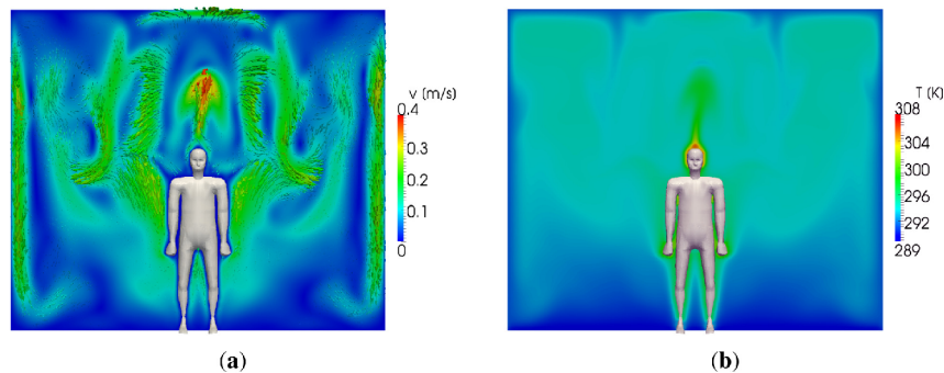
Obrázek 3.5: Mezní vrstva u lidského těla a) rychlostní pole b) teplotní pole (převzato z [15])
