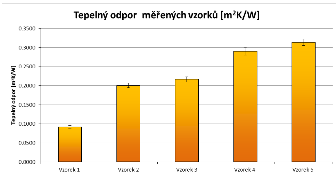
Obrázek 5.13: Graf tepelných odporů s nejistotami
