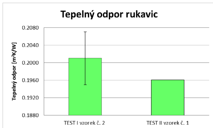
Obrázek 6.7: Porovnání výsledných tepelných odporů rukavic
