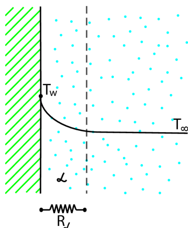
Obrázek 3.6: Přenos tepla mezní vrstvou při konvekci
