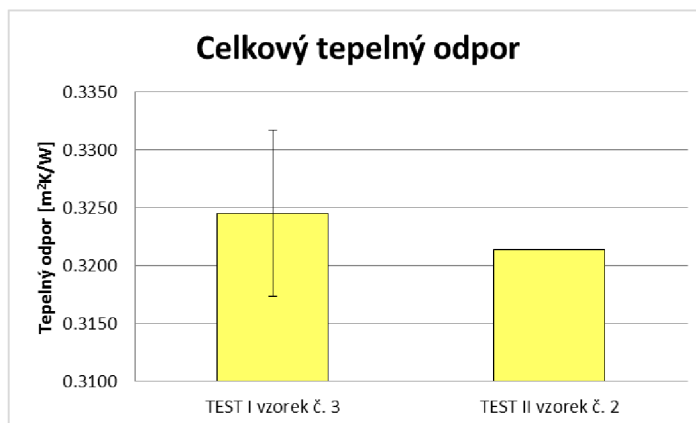
Obrázek 6.9: Porovnání celkových tepelných odporů
