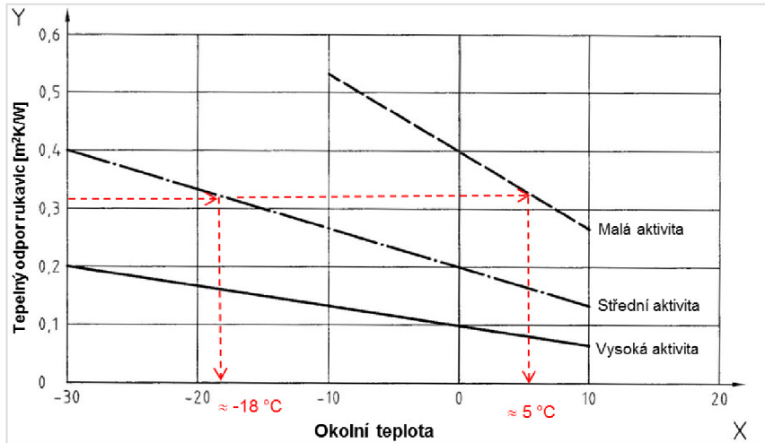
Obrázek 8.6: Graf pro určení použitelnosti vzorku č. 5
