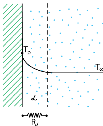
Obrázek 3.7: Přenos tepla mezní vrstvou při konvekcii
