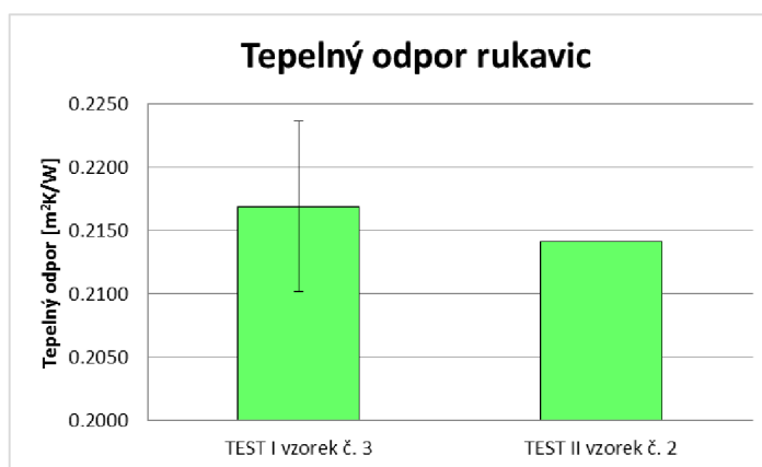
Obrázek 6.10: Porovnání výsledných tepelných odporů rukavic
