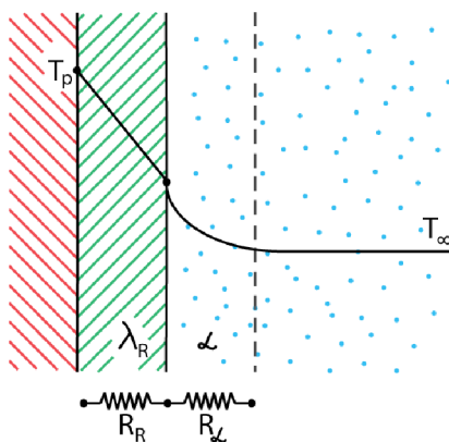
Obrázek 3.8: Vedení tepla přes rukavice
