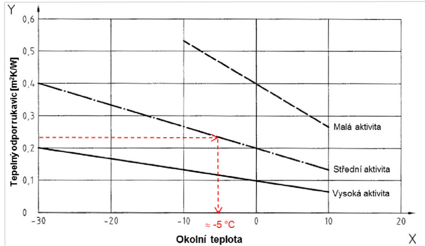
Obrázek 8.4: Graf pro určení použitelnosti vzorku č. 3
