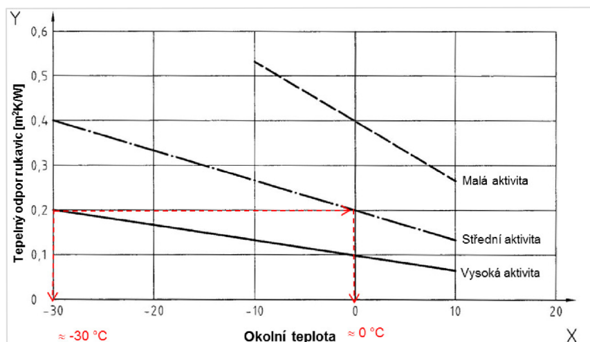
Obrázek 8.3: Graf pro určení použitelnosti vzorku č. 2
