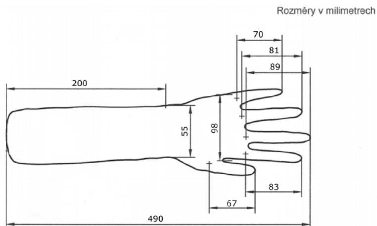
Obrázek 4.5: Rozměry Newtonovy ruky - upravený obrázek 4.4 podle naměřených rozměrů
