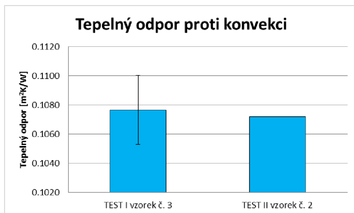
Obrázek 6.8: Porovnání tepelných odporů proti konvekci
