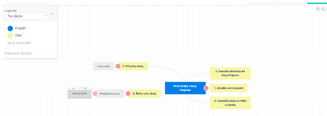
Obrázek 3.9: Vytváření WBS
