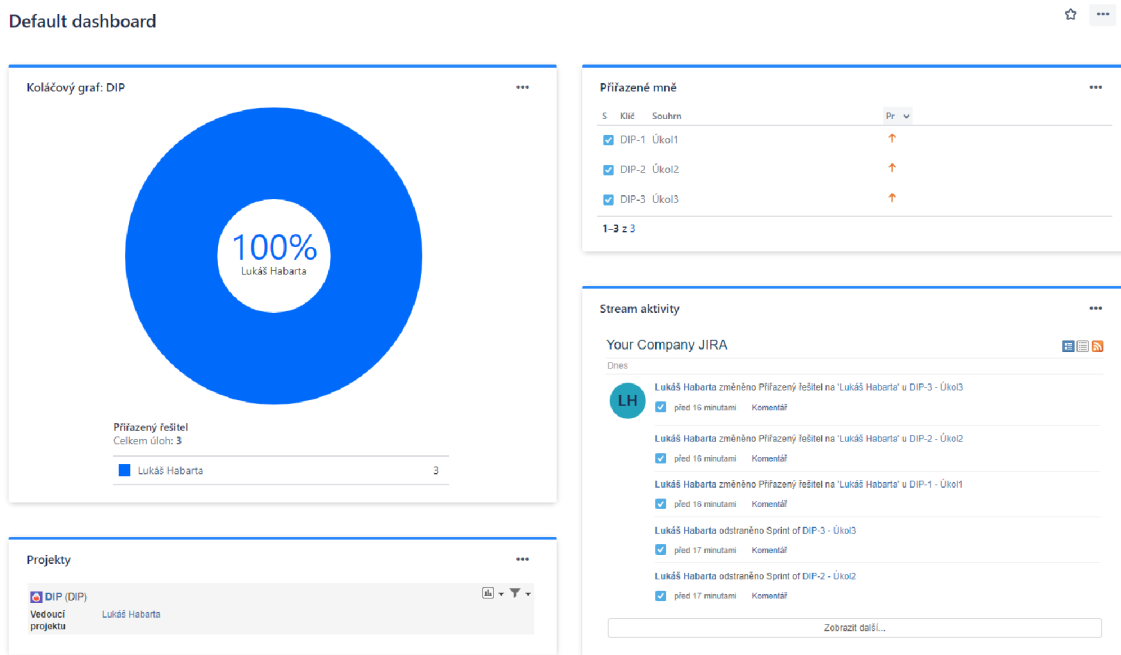
Obrázek 3.2: Dashboard
