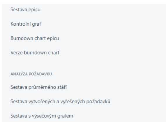
Obrázek 3.6: Výřez sestav
