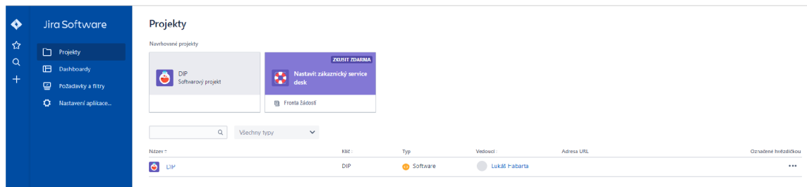
Obrázek 3.1: Přehled projektů.
