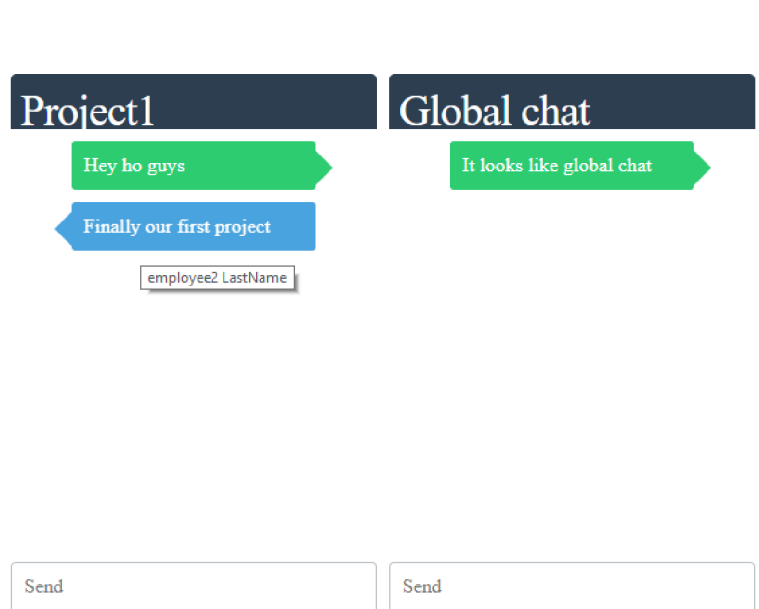
Obrázek 5.4: Chatovací rozhraní
