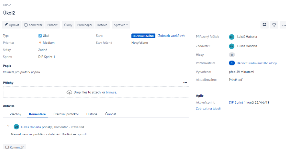
Obrázek 3.5: Detail úkolu
