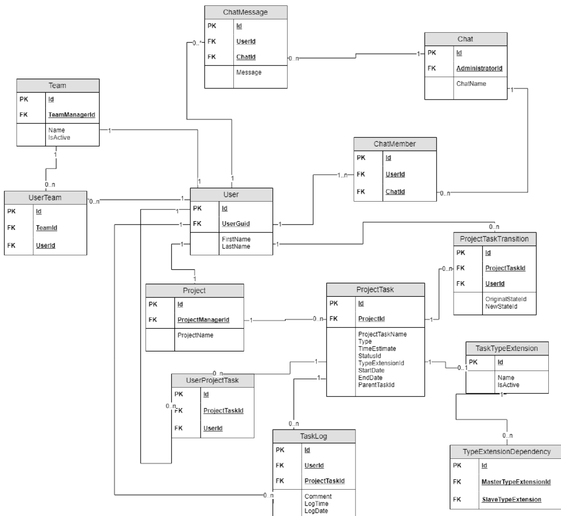
Obrázek 4.1: ER diagram
