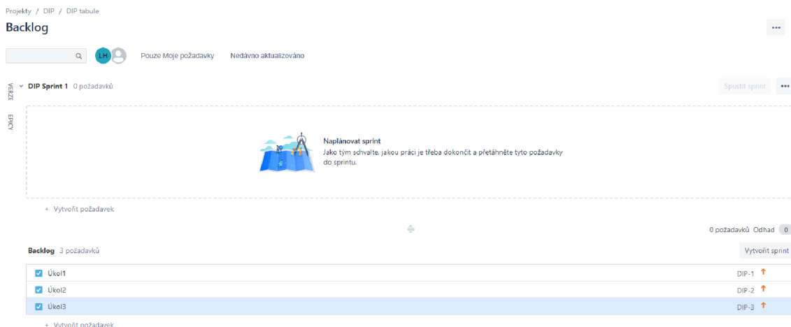
Obrázek 3.3: Detail projektu
