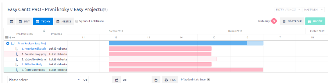
Obrázek 3.10: Ganttův diagram
