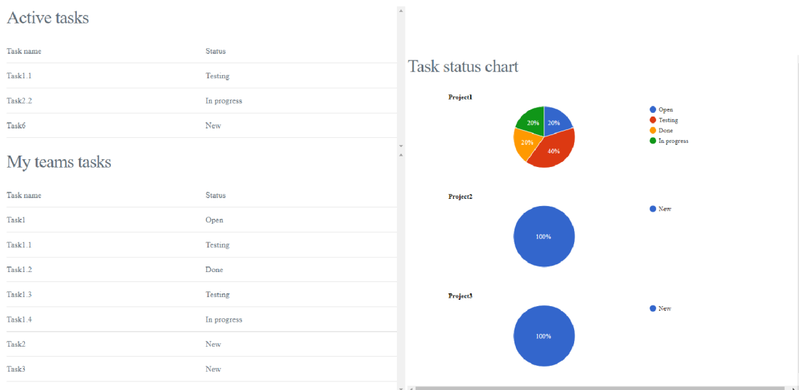
Obrázek 5.1: Dashboard stránka
