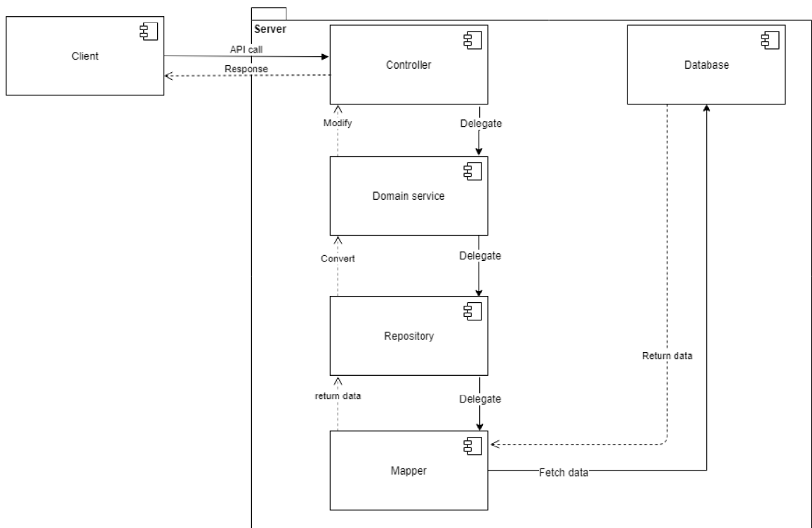
Obrázek 4.2: Nákres architektury a zpracování volání
