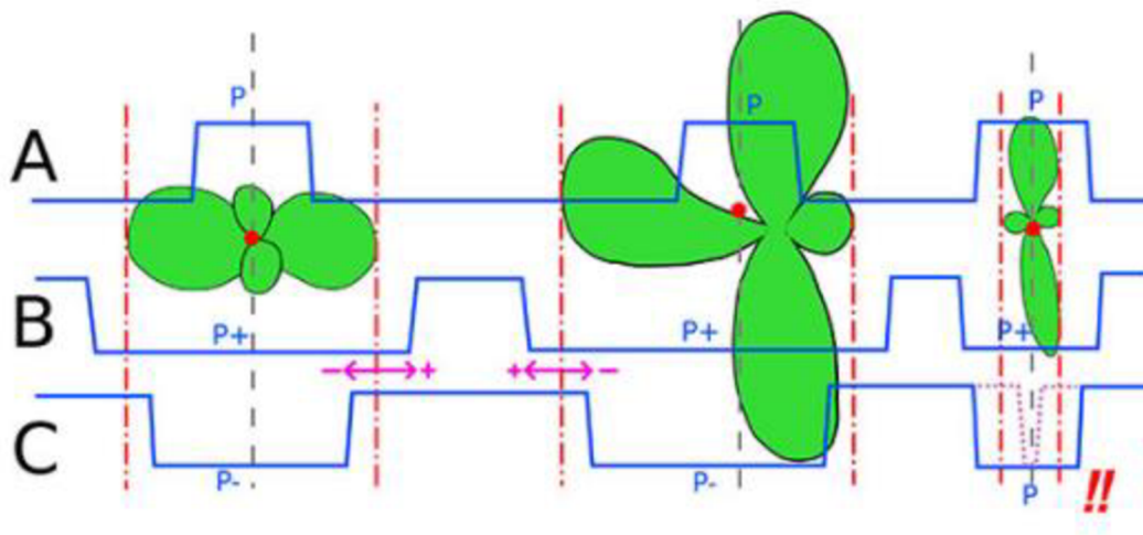
Obrázek 12: Dráha jednotlivých radliček v závislosti na nastavení systému
