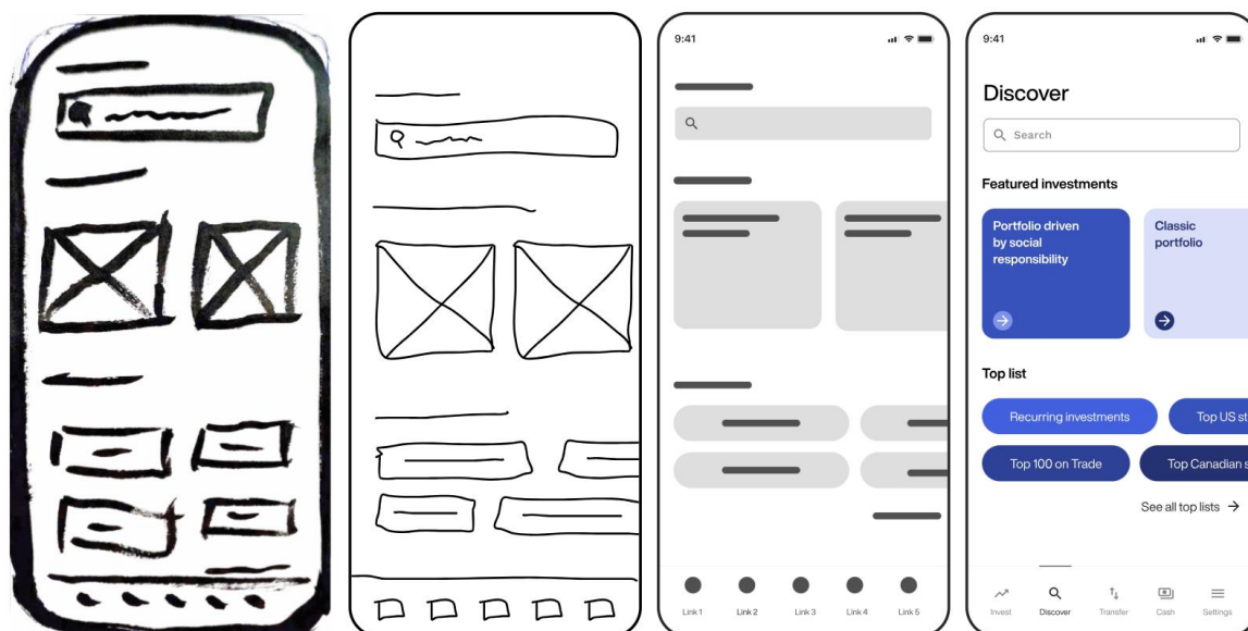
Obrázek 3 - Kategorie wireframů
