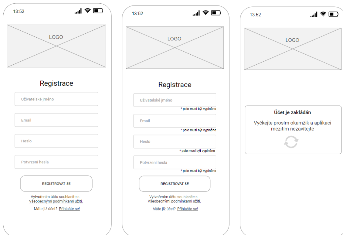
Obrázek 5 - Logický design – Registrace uživatele
