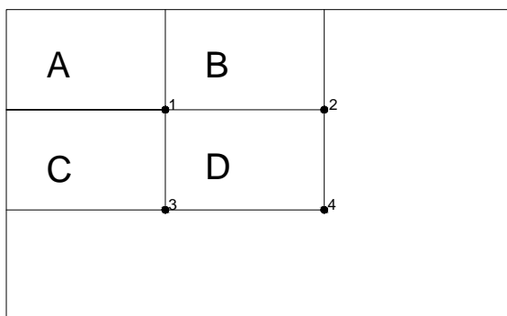
Obrázek 2.4: Příklad použití integrálního obrazu. Pokud bychom chtěli vypočítat součet hodnot všech pixelů pod písmenem D za pomoci integrálního obrazu, výpočet by vypadal takto: D_{sum} = s(4) + s(1) - (s(2) + s(3))
