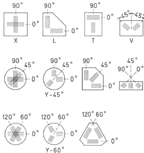
Obr.4.3 Tenzometrické růžice[7]
