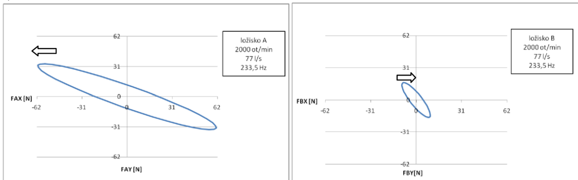
Graf. 4.22 U ložiska A dochází k protiběžné precеси, u ložiska B k souběžné precеси
