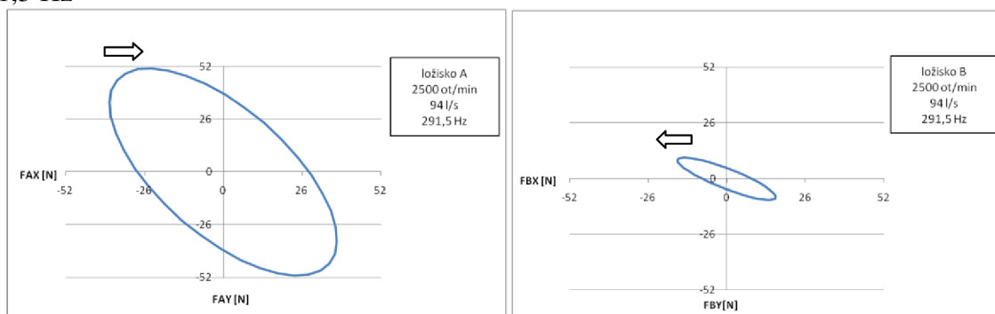
Graf. 4.32 U ložiska A dochází k souběžné precisi, u ložiska B k protiběžné precisi
