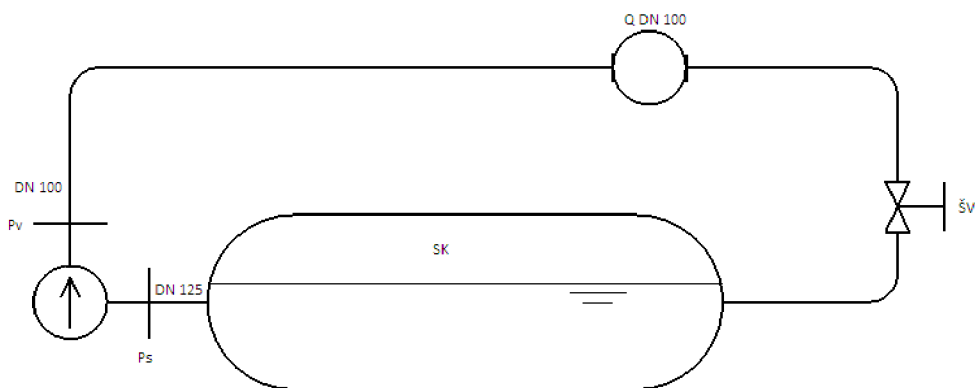
Obr. 2.2 Měřicí trať
