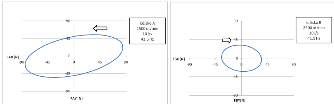
Graf. 4.23 U ložiska A dochází k protiběžné precеси, u ložiska B k souběžné precеси
