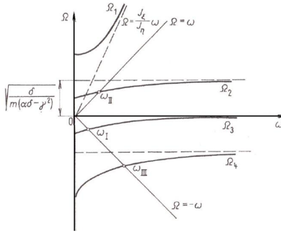
Obr. 3.5 Závislost kořenů rovnice 2.40 na úhlové rychlosti \omega . [6]
