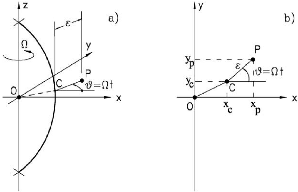
Obr. 3.3 Nevyvážený Lavalův rotor s nevyvážkou m\varepsilon . (a) Nákres soustavy. (b) Stav v rovině xy . [6]
