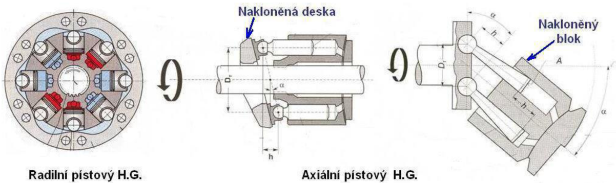
Obr. 1.2 Schéma radiálních a axiálních pístových čerpadel [1]
