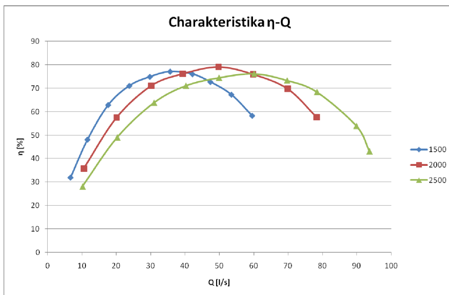
Graf 4.3 Závislost účinnosti na průtoku
