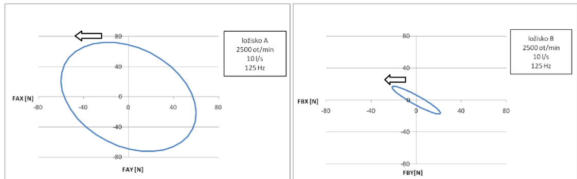
Graf. 4.24 Zde dochází k protiběžné precеси
