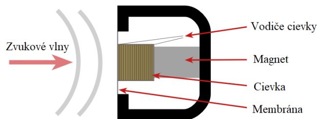
Obr. 2.4: Štruktúra dynamického mikrofónu [6]
