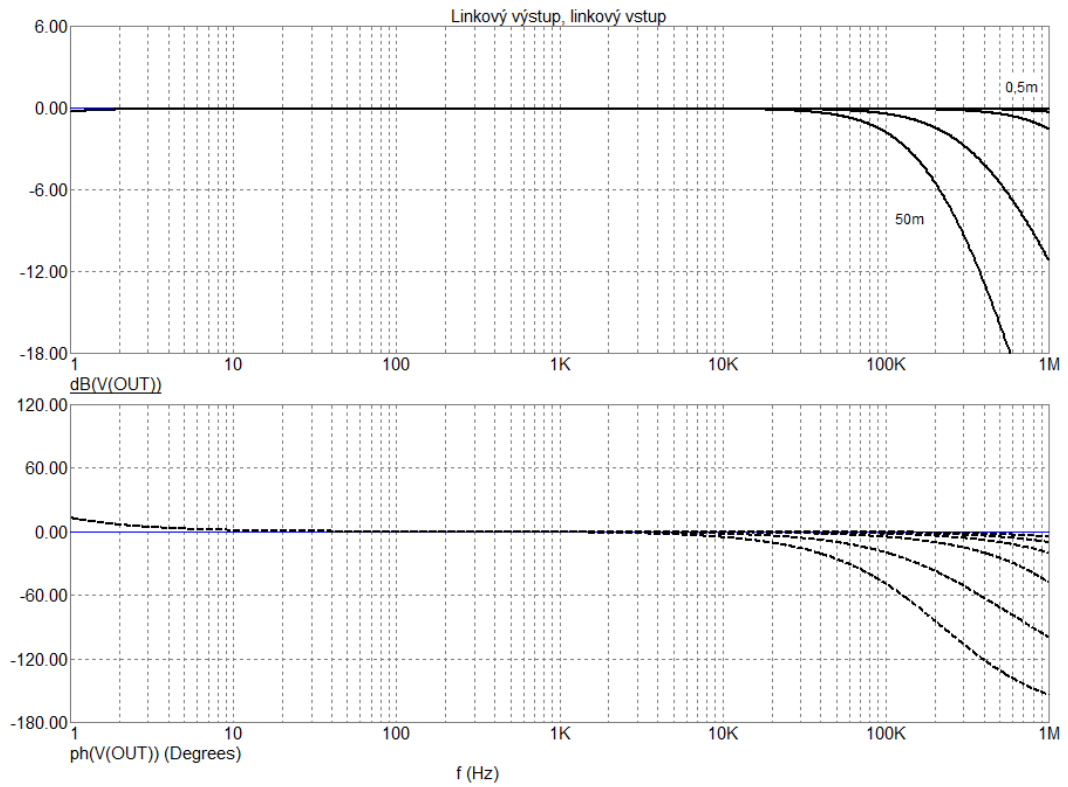
Obr. 3.12: Graf lineárneho skreslenia zapojenia linkový výstup - linkový vstup, 6300FH
