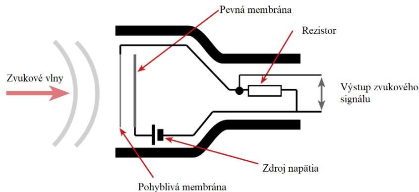
Obr. 2.6: Štruktúra kondenzátorového mikrofónu [8]
