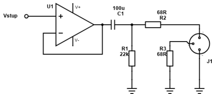
Obr. 2.9: Schéma zapojenia linkového výstupu [1]
