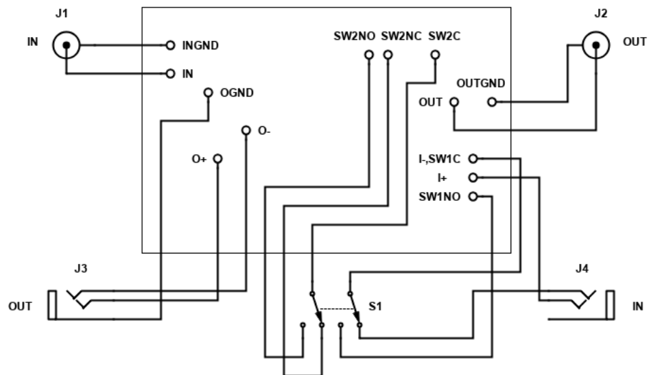
Obr. 4.11: Blokova schéma pripojenia prepínača SYM/NESYM a konektorov do DPS
