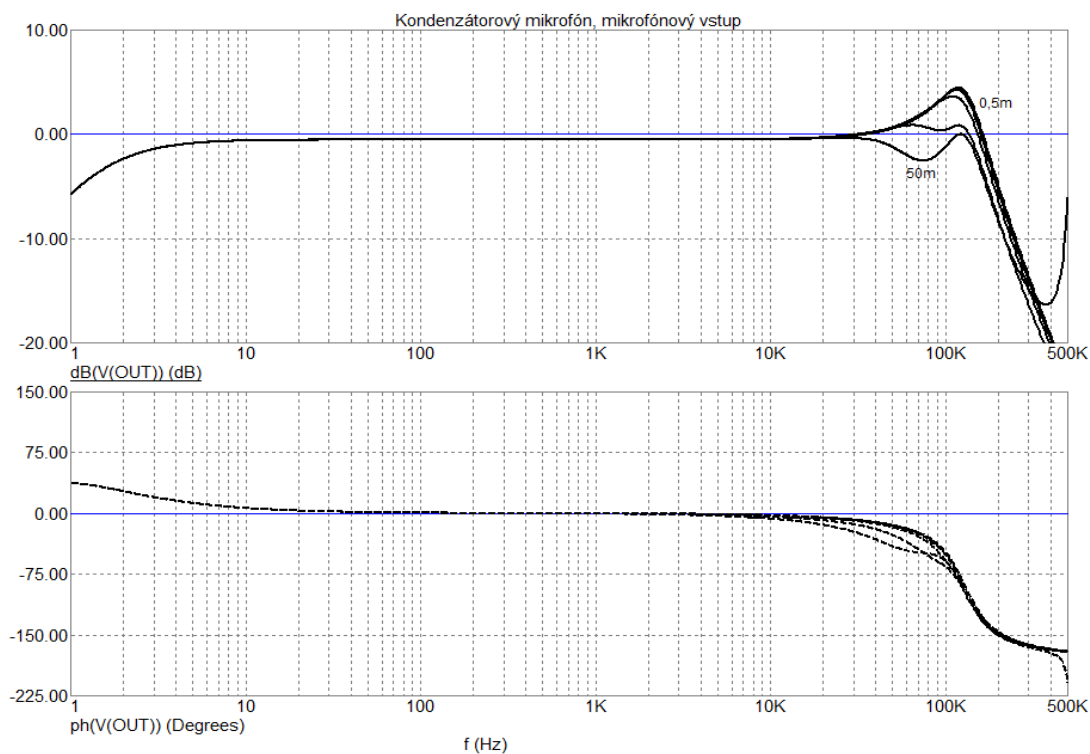
Obr. 3.6: Graf lineárneho skreslenia zapojenia kondenzátorový mikrofón – mikrofónový vstup, kábel 6300FH
