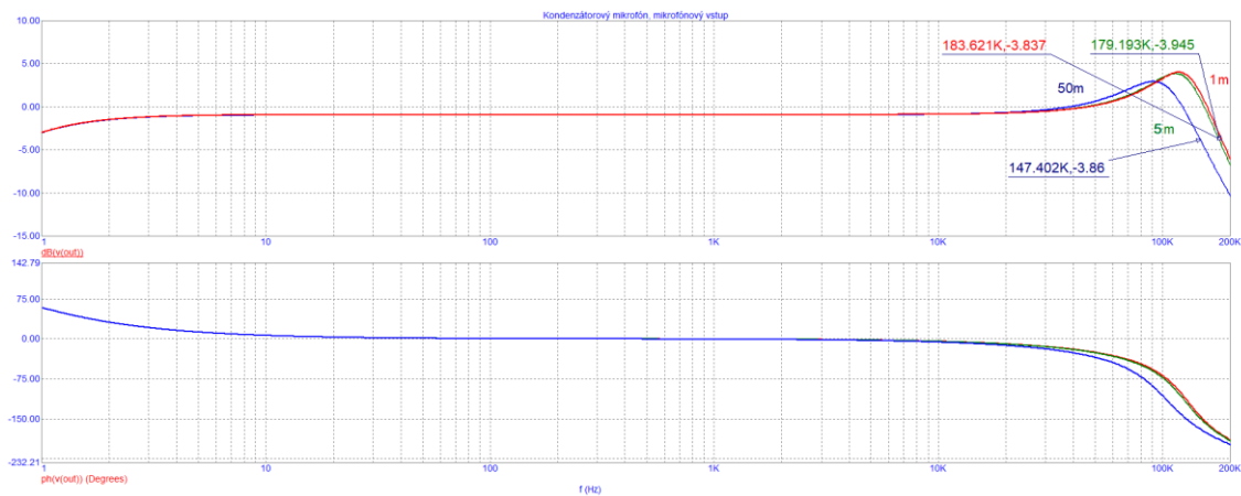
Obr. 4.6: Graf lineárneho skreslenia simulácie zapojenia kondenzátorový mikrofón – mikrofónový vstup
