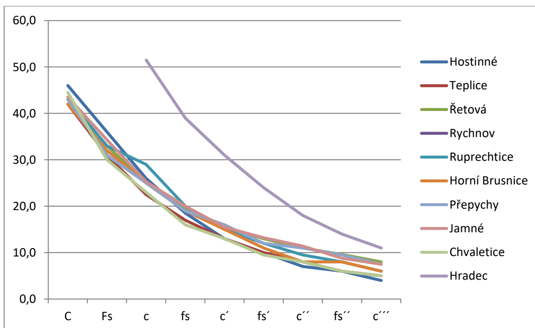
Tabulka č. 32 – porovnání menzur restřiku Oktáva 2' (Octava 2', Superoctava 2')
