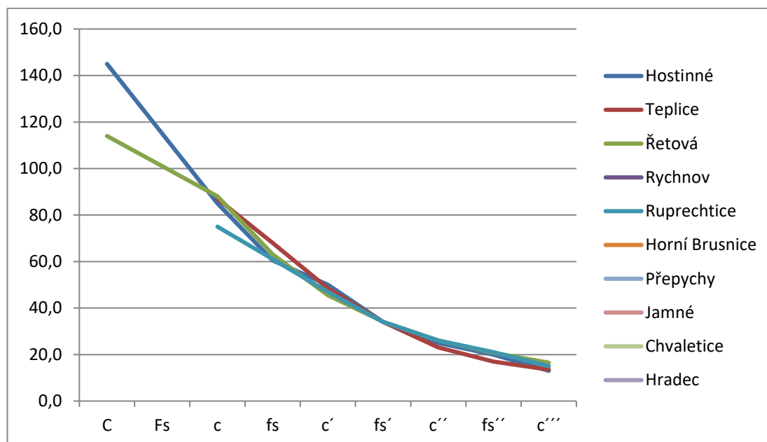
Tabulka č. 29 – porovnání menzur restříku Principál 8'
