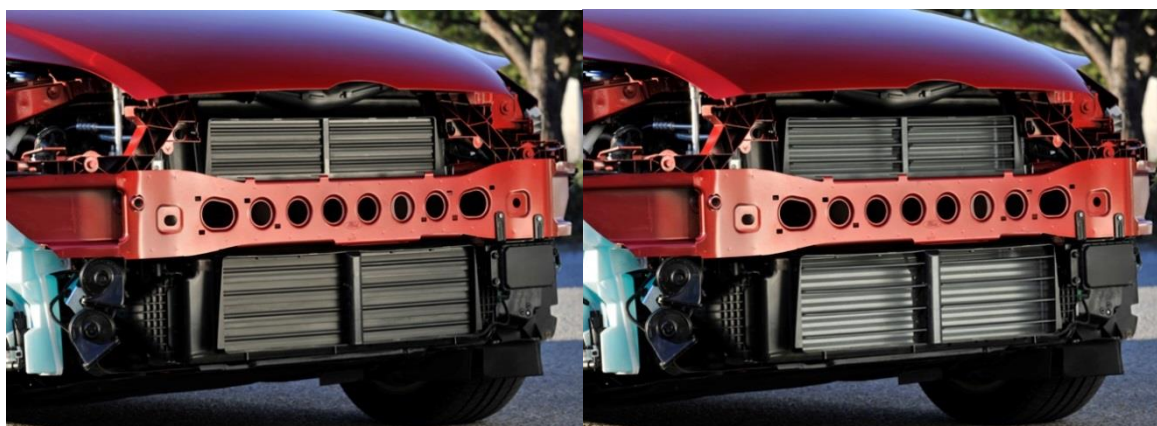
Obr. 33 Uzavřené klapky (vlevo) a otevřené klapky (vpravo) na voze Ford Focus [3]
