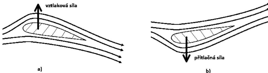
Obr. 2 Profil křídla a) letadla, b) automobilu [12]
