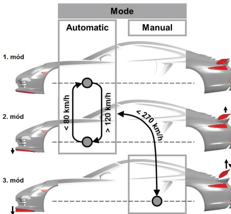
Obr. 30 Strategie přepínání mezi módy u vozu Porsche 911 Turbo S [2]
