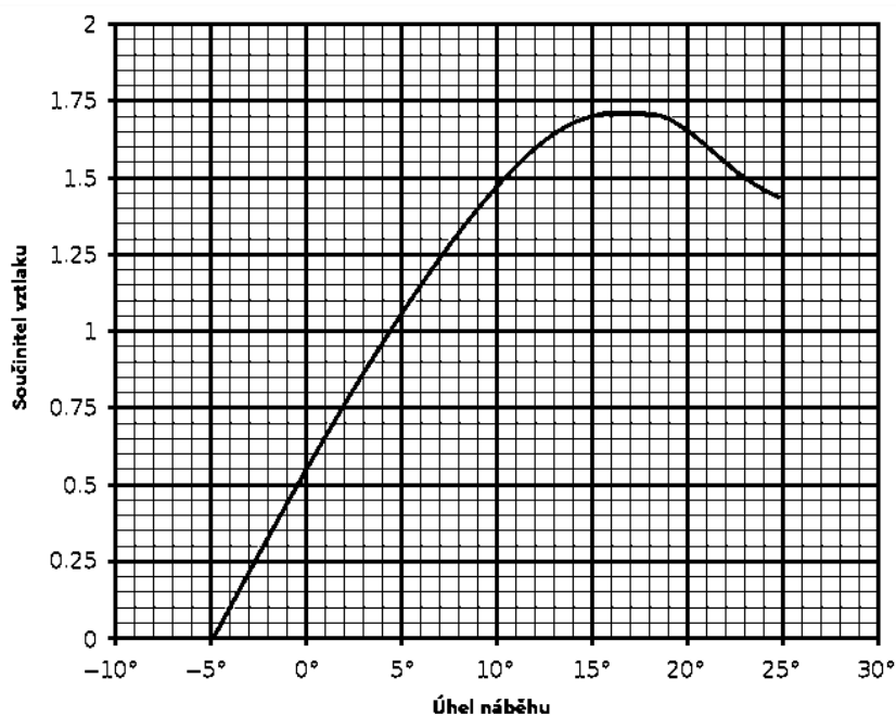
Obr. 4 Závislost vztlaku a úhlu náběhu u leteckého křídla [6]
