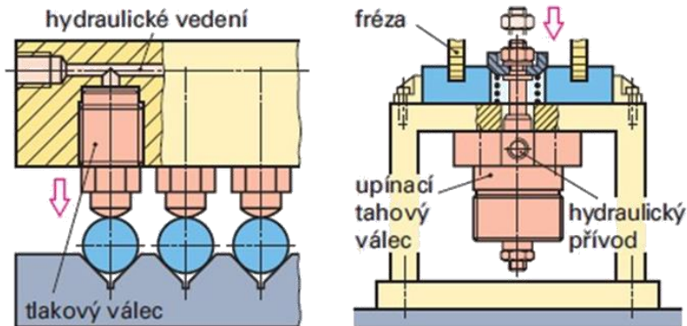
Obr. 18) Hydraulické upínací přípravky [11]
