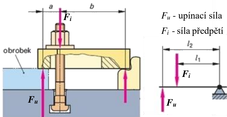
Obr. 33) Znázornění sil působıcıch na upınkou [11]
