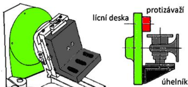
Obr. 8) Upínací úhelník [7]
