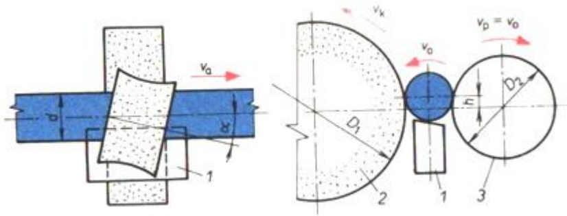
Obr. 21) Bezhruté broušení vnějších válcových ploch. 1) Podpěrné pravítko, 2) Brusný kotouč, 3) Unášecí kotouč [2]
