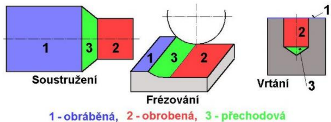
Obr. 1) Vytvořené plochy při obrábění na obrobku [1]
