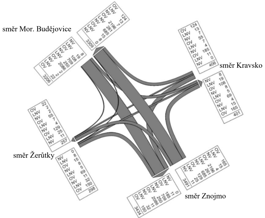
Obrázek 9 - Pentlogram stávající křižovatky I/38 a III/40826
