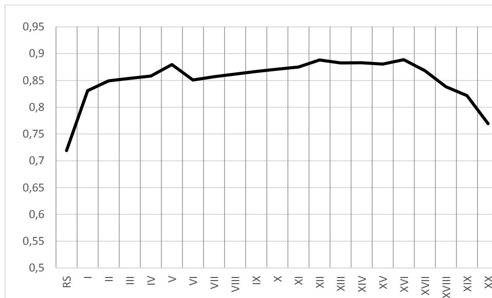
Obrázek 8.1 Účinnost jednotlivých stupňů, včetně regulačního
