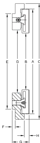
Obrázek 7.2 Rozměry axiálního ložiska, převzato z [8]
