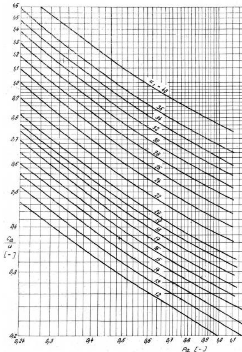
Obrázek 3.1 Diagram pro výpočet skupiny přetlakových stupňů metodou \frac{c_a}{u} , převzato z [1]
