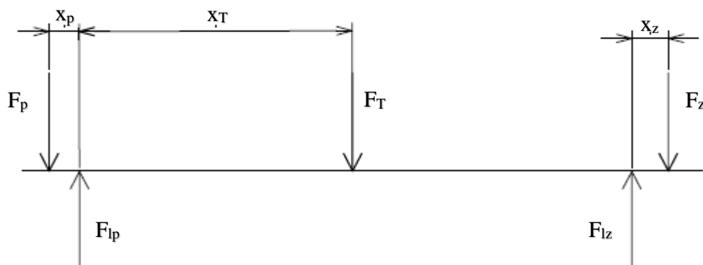
Obrázek 7.3 Znáornění rozložení sil nesených radiálním ložiskem
