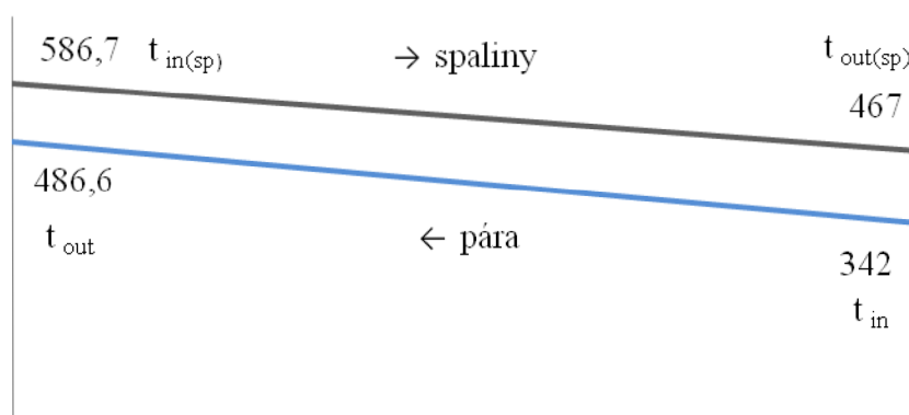
Obr. 13 Teplotní spád přihříváku RH 1
