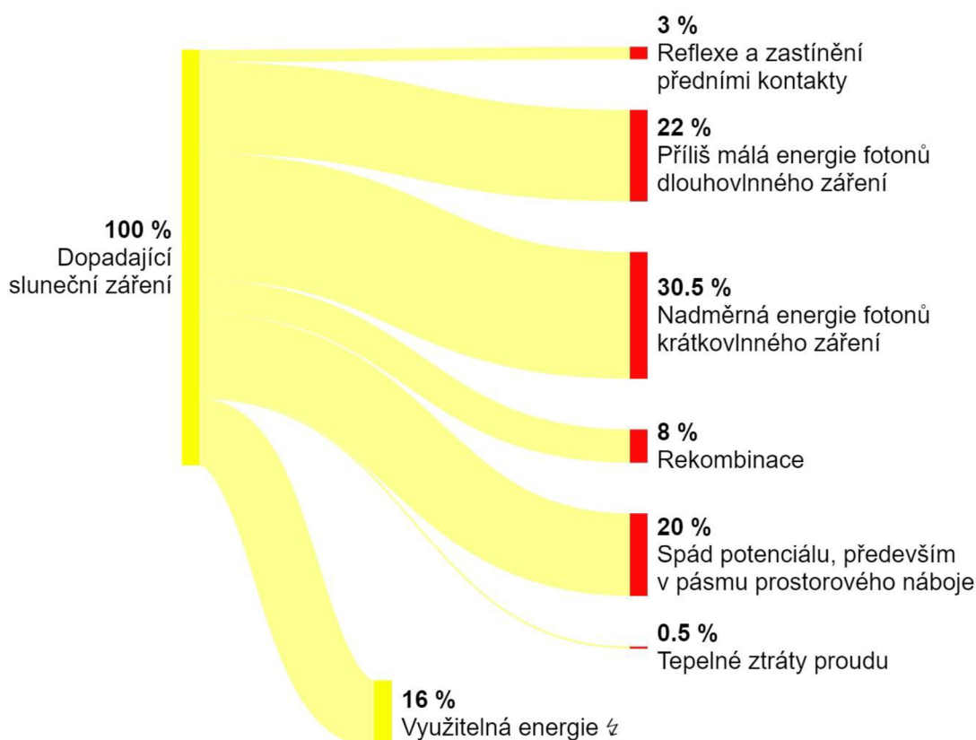
Obr. 5 Diagram toku energie dopadající na solární článek (převzato a upraveno z [8])
