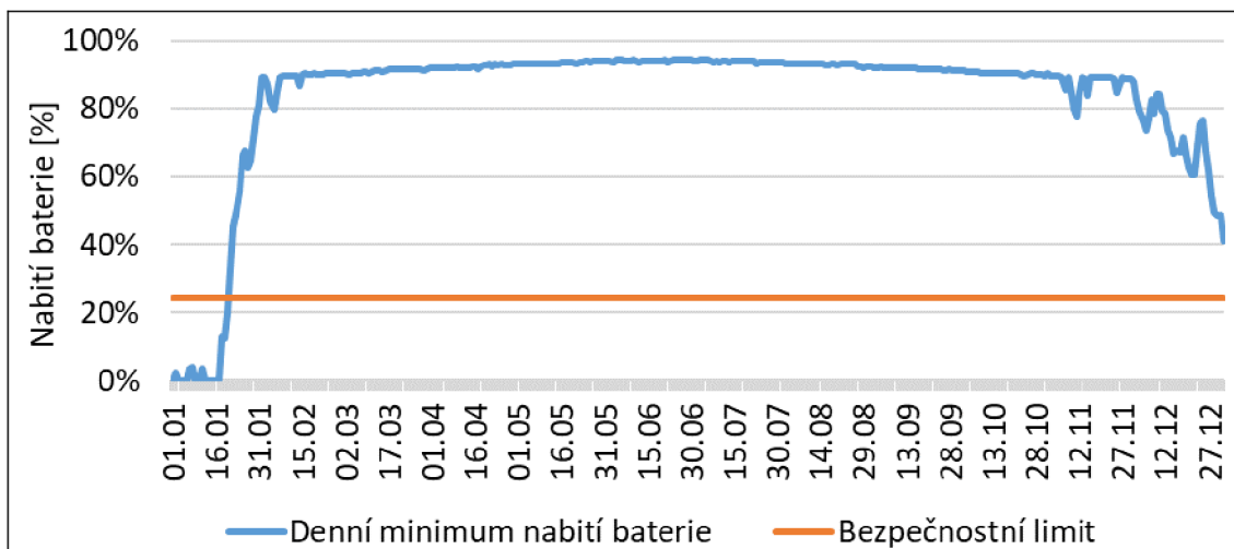
Obr. 54 Průběh min. denních kapacit u PV systému v konfiguraci M9-3-3-1999
