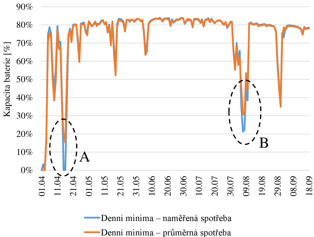
Obr. 45 Porovnání minimálních denních hodnot použitím původních dat spotřeby a jejich průměru (konfigurace 1-1)
