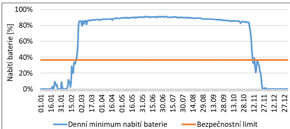
Obr. 53 Průběh min. denních kapacit u PV systému v konfiguraci M9-2-2-1999
