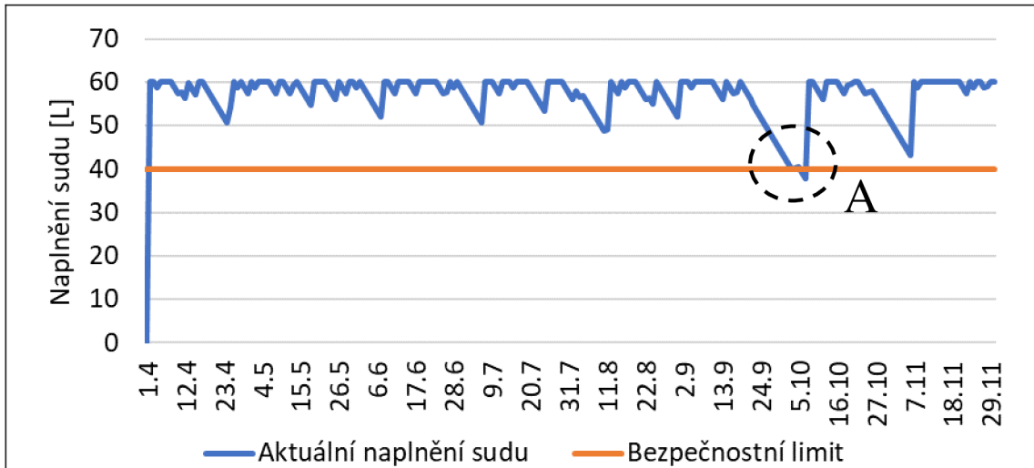
Obr. 56 Průběh denních kapacit u závlahového systému v konfiguraci L6–60L–2015 s vyznačením podlimitní kapacity
