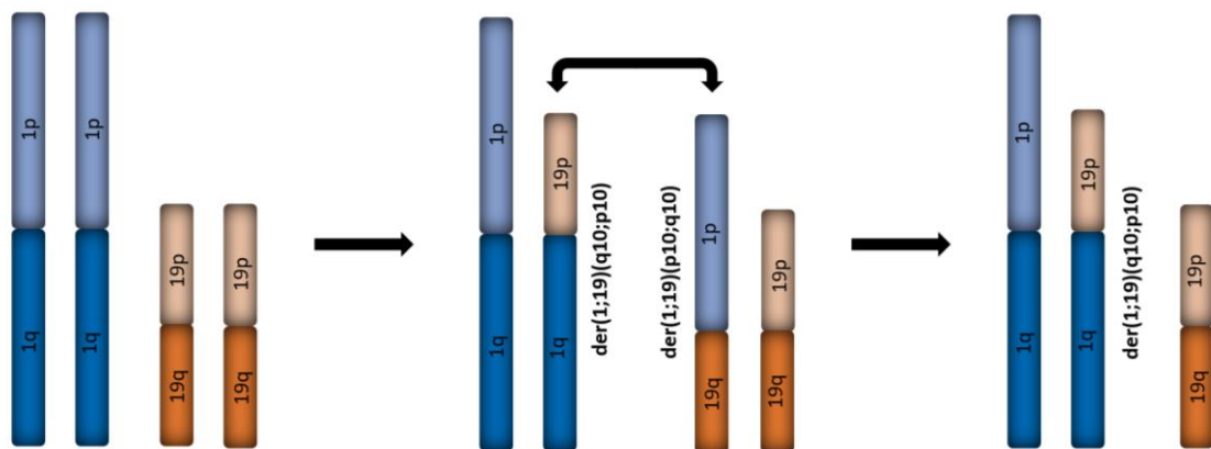
Obr. 1: Mechanismus chromozomové kodelece ramen 1p/19q u Oligodendrogliomu, IDH-mutant s kodecí 1p/19q (převzato a upraveno dle Griffin et al., 2006)
