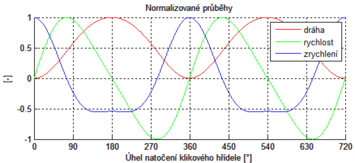
Obr. 30 Normalizované průběhy dráhy, rychlosti a zrychlení v závislosti na natočení klikového hřídele pro 6\,500\text{ min}^{-1}
