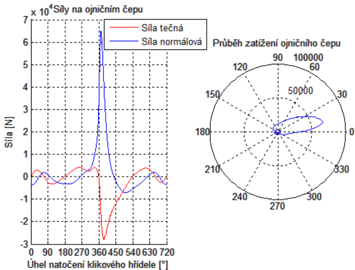
Obr. 43 Síly působící na ojnicím čepu
