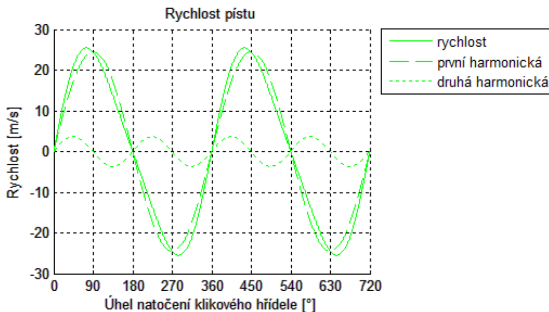
Obr. 28 Závislost rychlostí pístu na úhlu natočení klikového hřídele pro 6 500 min -1
