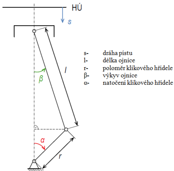
Obr. 26 Dráha pístu [15]
