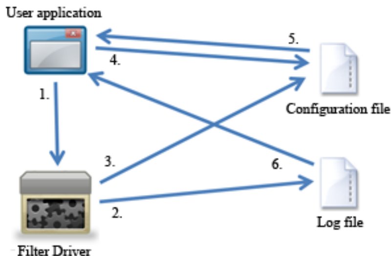
Obrázok 6: Dátový tok v Personal DLP.
