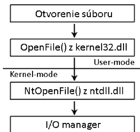
Obrázok 4: Činnosť operačného systému pri otváranie súboru.
