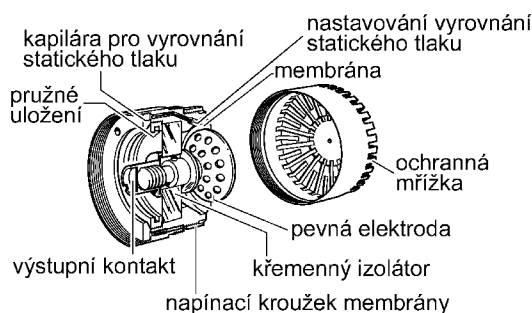
Obr. 1 Řez mikrofonom B&K [43]
