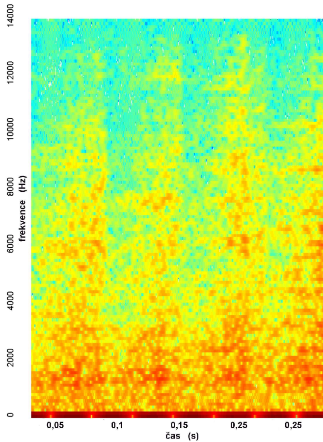
Obr. 17 Časově frekvenční analýza hluku motoru
