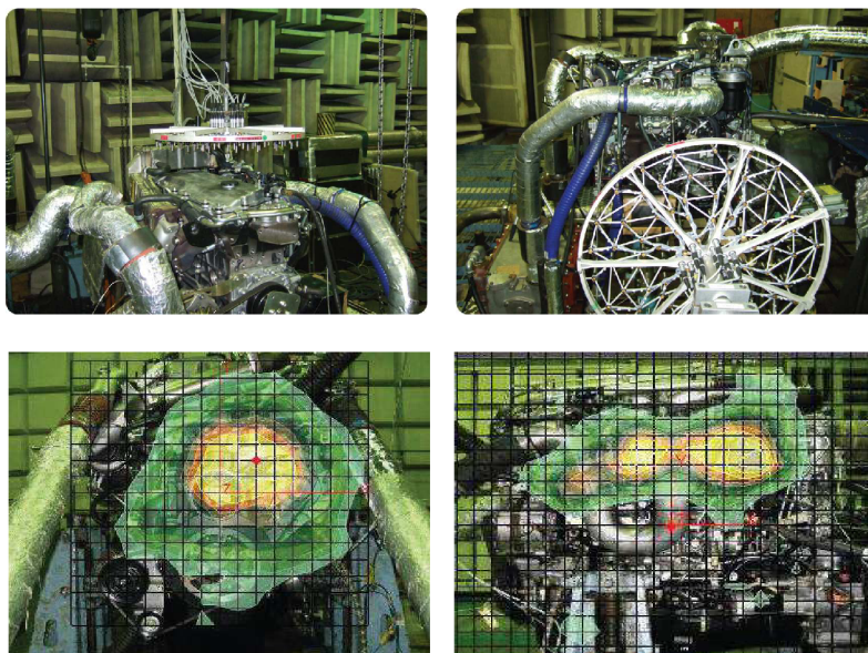
Obr. 21 Akustická holografie v blízkém poli [48]
