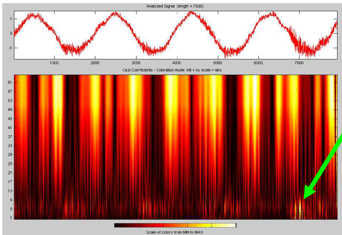
Obr. 15 Zpracování signálu spojitou vlnkovou transformací (vlnka typu gaus, 1. řád)
