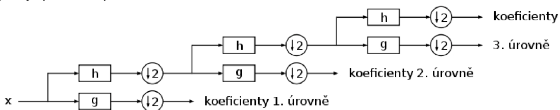
Obr. 10 Banka filtrů diskretní vlnkové transformace
