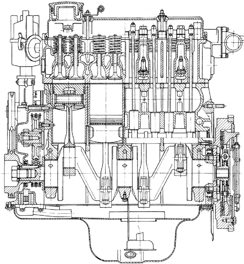
Obr. 56 Řez motorem Škoda [2]
