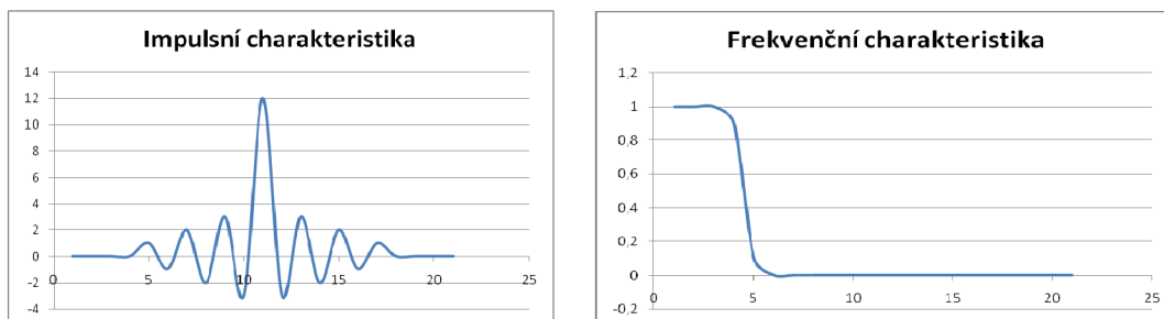
Obr. 8 Impulsní a frekvenční charakteristika lineárního filtru
