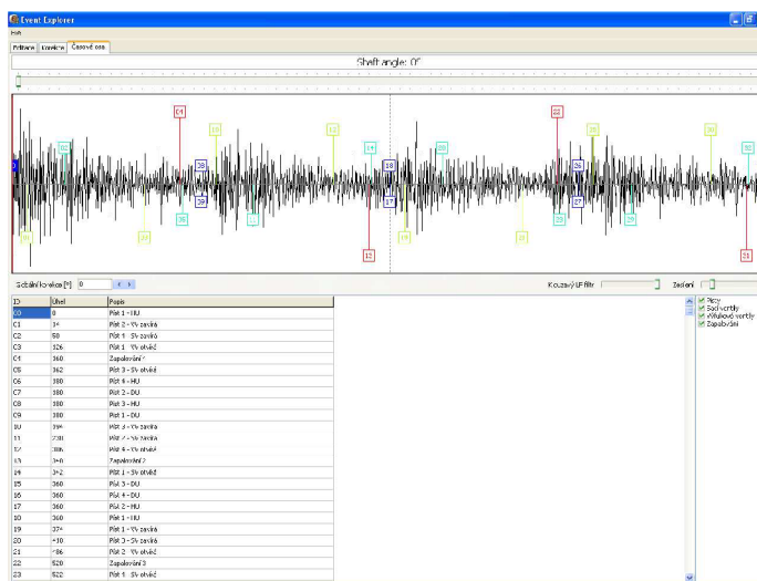
Obr. 54 Diagram událostí s upraveným časovým záznamem hluku motoru
