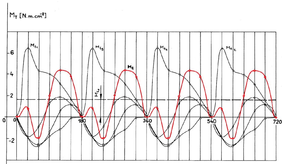
Obr. 33 Průběh točivého momentu čtyřválcového motoru před setrvačником [25]
