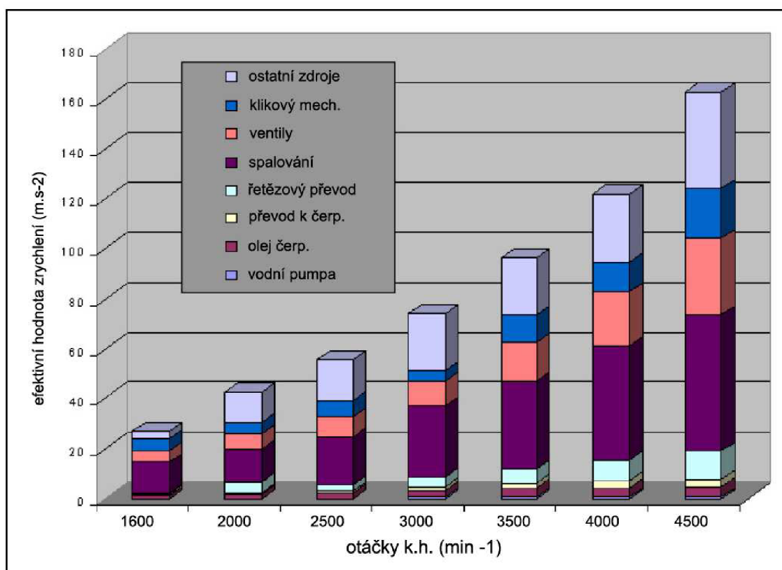
Obr. 19 Porovnání vibrační zdrojů, maximální točivý moment [11]
