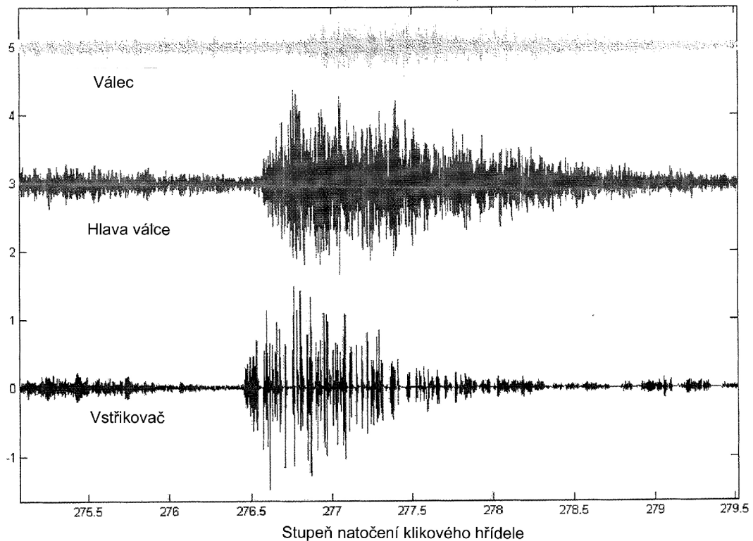
Obr. 41 Záznam vibrací stejného zdroje (vstřikovače) na různých místech motoru [24]
