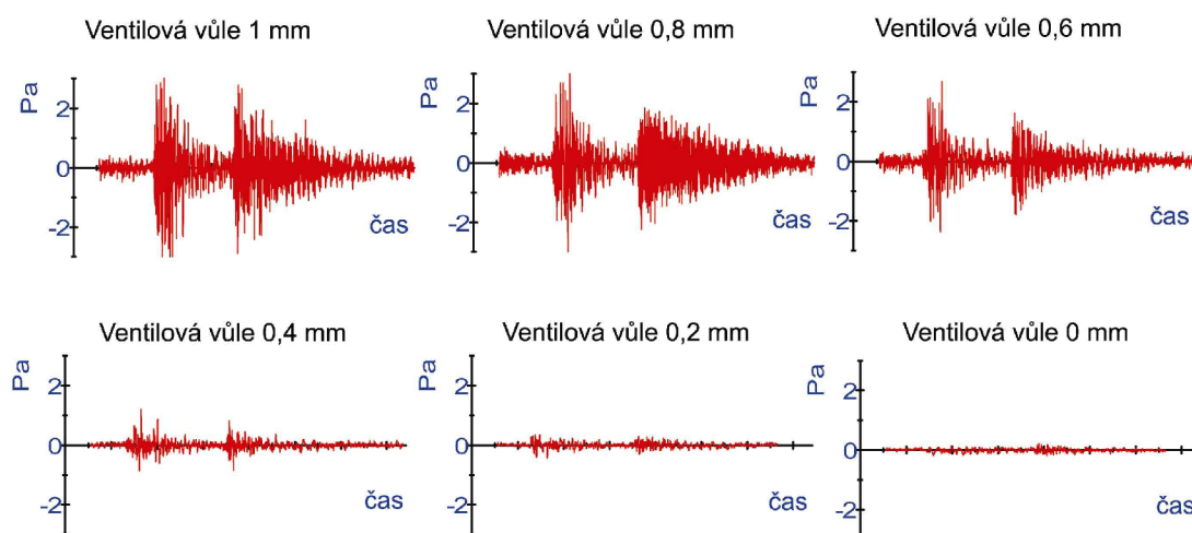
Obr. 47 Vliv ventilové vůle na hluk rozvodového mechanismu
