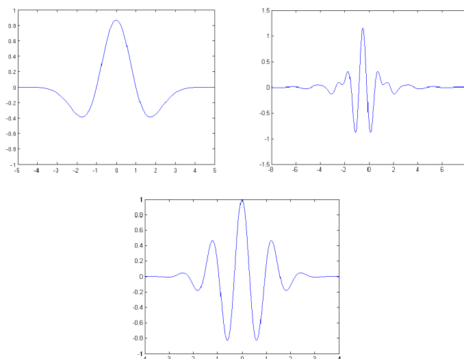
Obr. 12 Typy vlnek pro diskretní vlnkovou transformaci: Mexická, Morlet, Meyer
