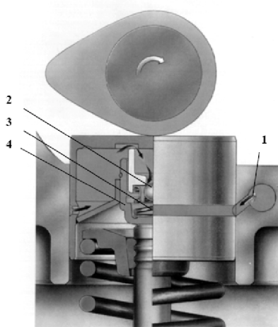
Obr. 27 Hydraulický vmezovač vůle hrníčkovým zdvihátkem [44]
