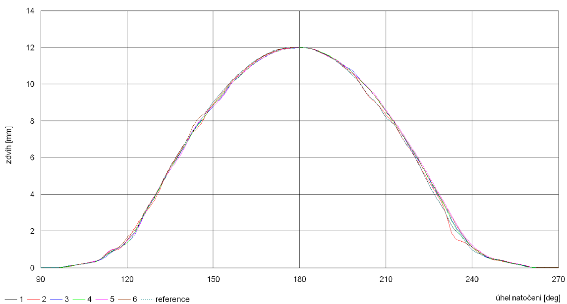
Obr. 31 Porovnání palců vačky u šestiválcového motoru sportovního vozu (2). [32]
