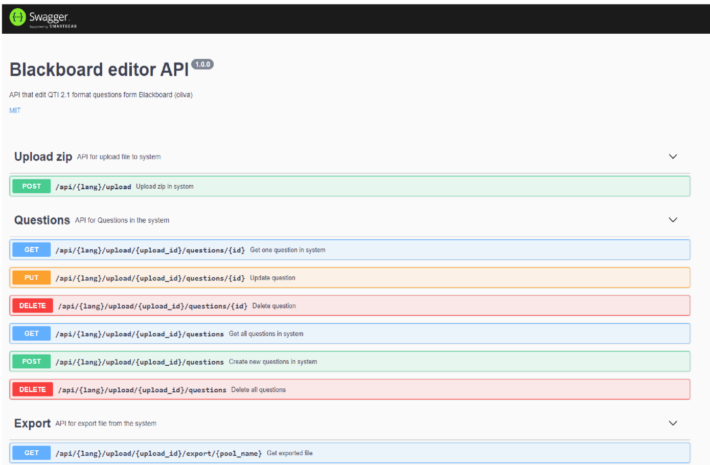
Obr. 8 Zobrazení Swagger dokumentace
