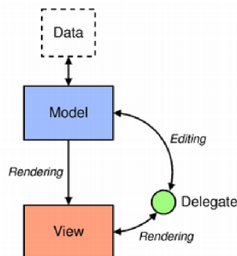
Obrázek 6.6: Model/View architektura
