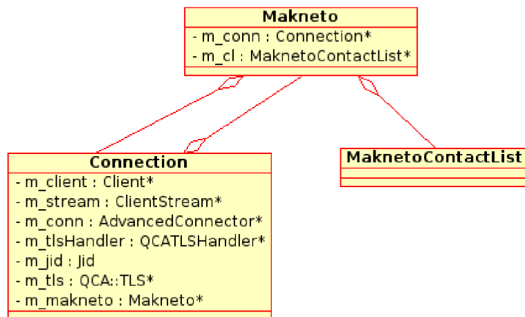
Obrázek 6.2: Diagram tříd Makneto
