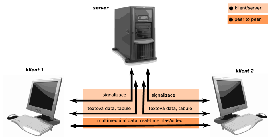
Obrázek 4.1: Návrh architektury
