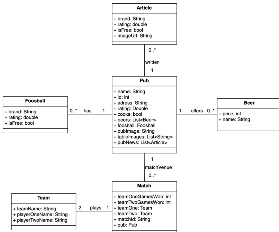
Obrázek 19 Diagram tříd
