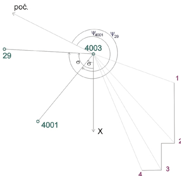
Obr. 6: Polárna metóda [21]
