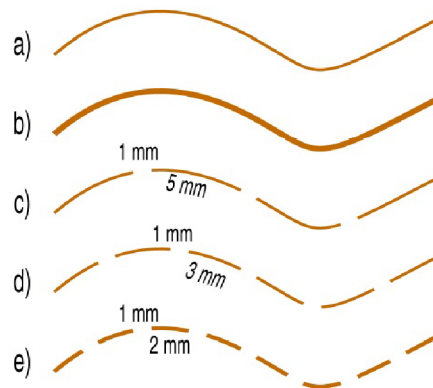
Obr. 2: Znáozornenie vrstevníc
