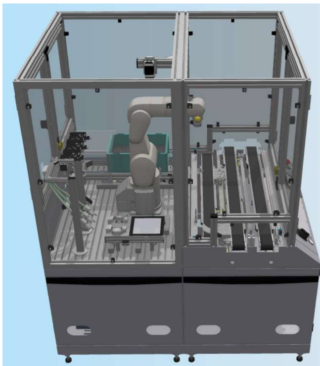
Obr. 9: Moduly buňky a) víceúrovňový sklad, b) robotická osazovací buňka [13]
