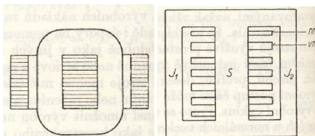
Obr. 5.1-2 Plášťové transformátory[1]
