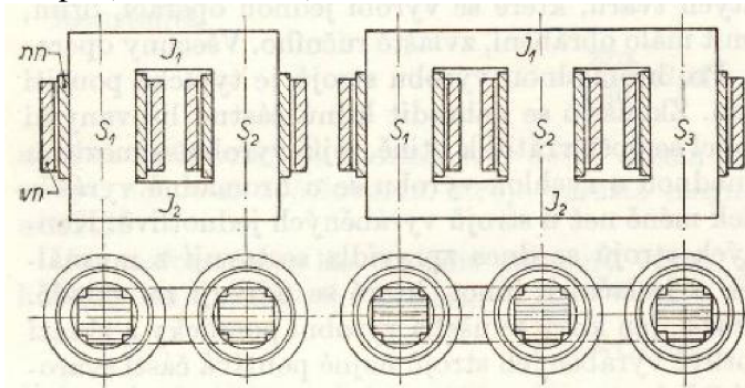
Obr.5.1-1 Jádrové transformátory[1]
