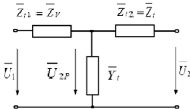
Obr. 6-3 Náhradní schéma vedení a transformátoru nesouměrným T člunkem
