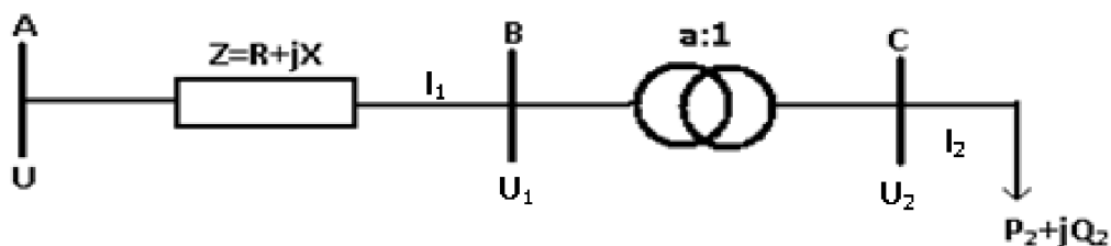
Obr. 5.5-1 Zjednodušené schéma distribuční sítě
