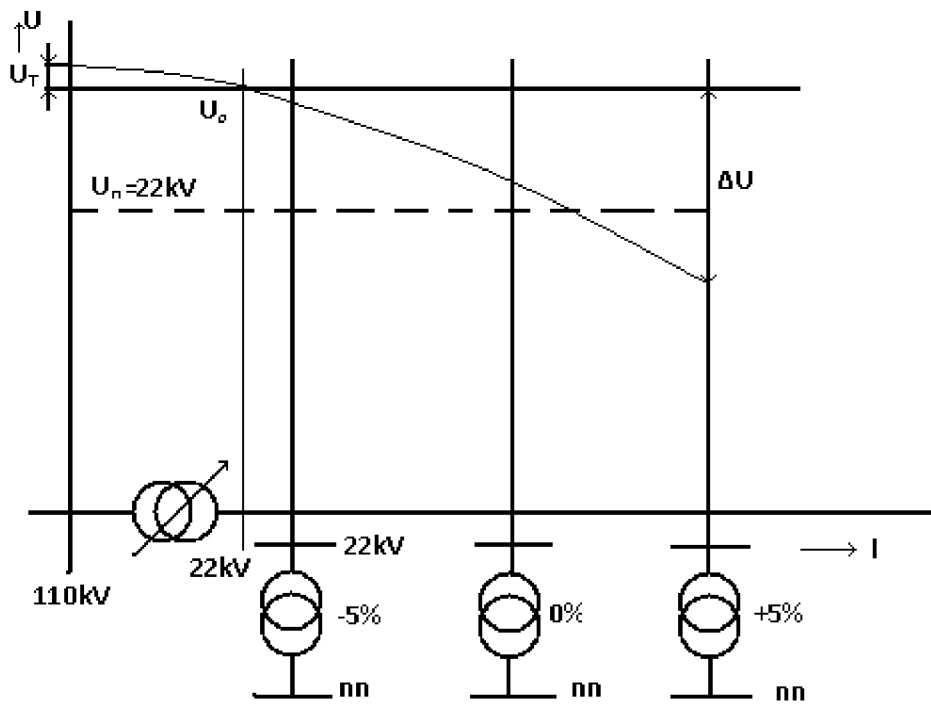
Obr. 5.5-4 Princip regulace napětí v distribučních sítích
