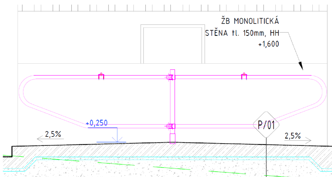
Obrázek 20 - Výkresový řez-lehací boxy ( Koblíška, 2023)
