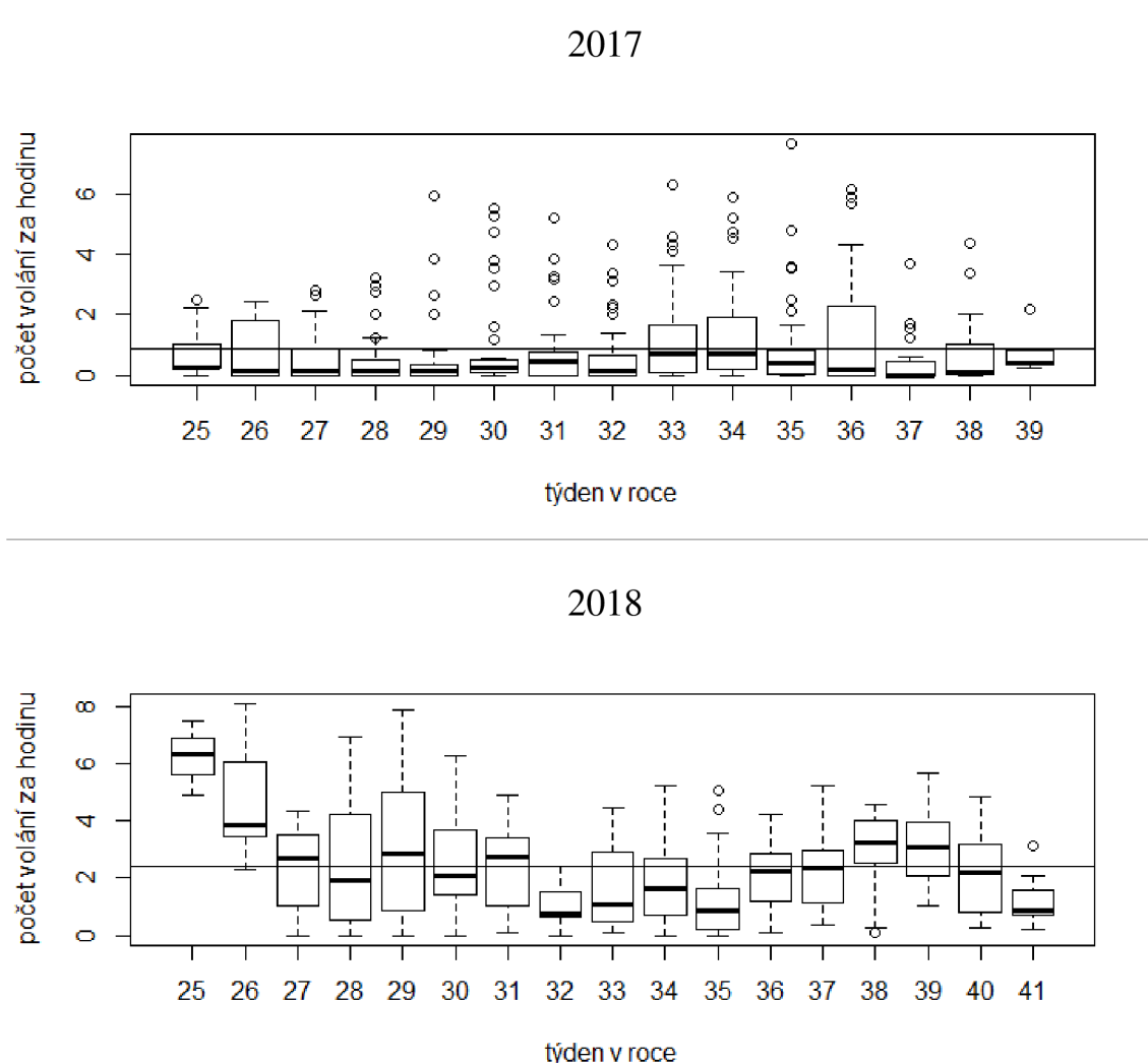
Obrázek 8 Box plot počtu volání za hodinu v jednotlivých týdnech v sezóně. Přímka zobrazuje průměrnou hodnotu počtu volání za hodinu ( 0,87 \pm 1,38 v roce 2017 a 2,40 \pm 1,85 v roce 2018).
