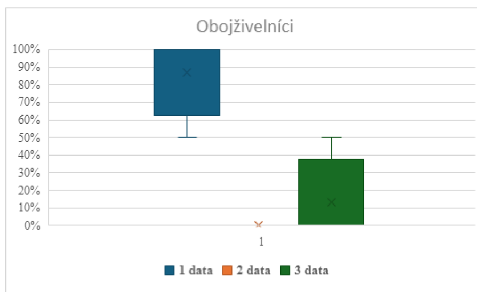
Graf 4.4: Typy dat pro obojživelníky - krabicový graf (průměr, kvartily a min-max)
