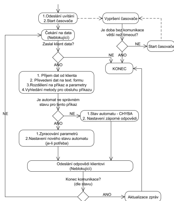
Obrázek 9.4: Schéma práce třídy Pop3Handler
