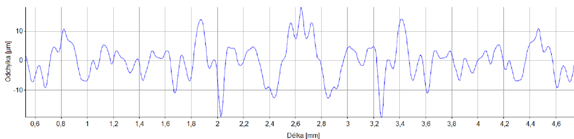
Obr. 4.50 Vyhodnocená drsnost při n = 3000 \text{ min}^{-1} a f = 0,05 \text{ mm} .
