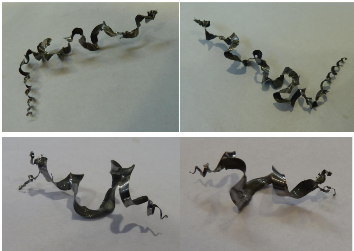
Obr. 4.46 Ukázka dlouhých třísek.
