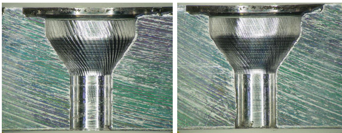
Obr. 4.47 Znehodnocený povrch otvoru.
