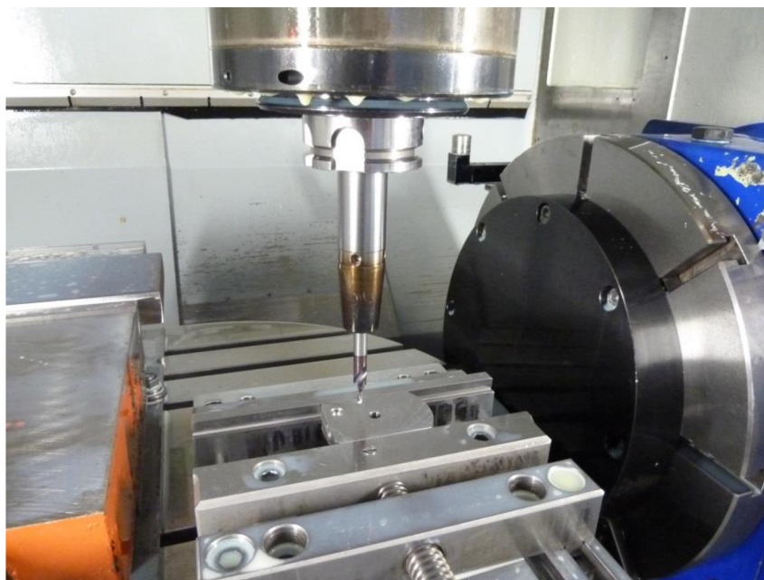
Obr. 4.29 Nastavení experimentálního obrábění.
