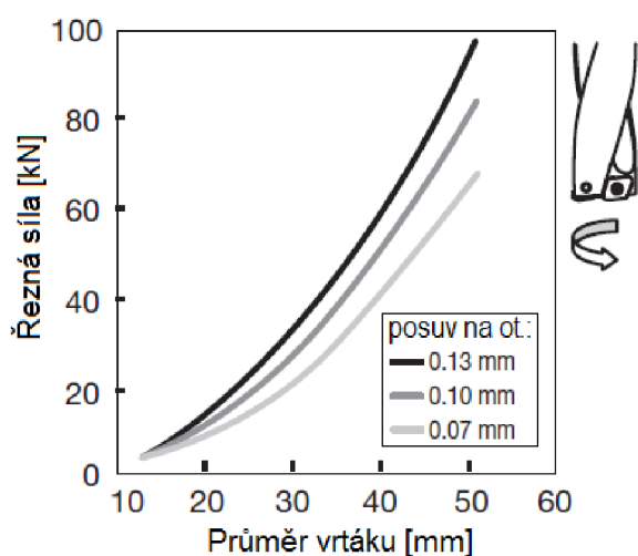
Obr. 1.10 Závislost řezné síly na průměru vrtáku [9].
