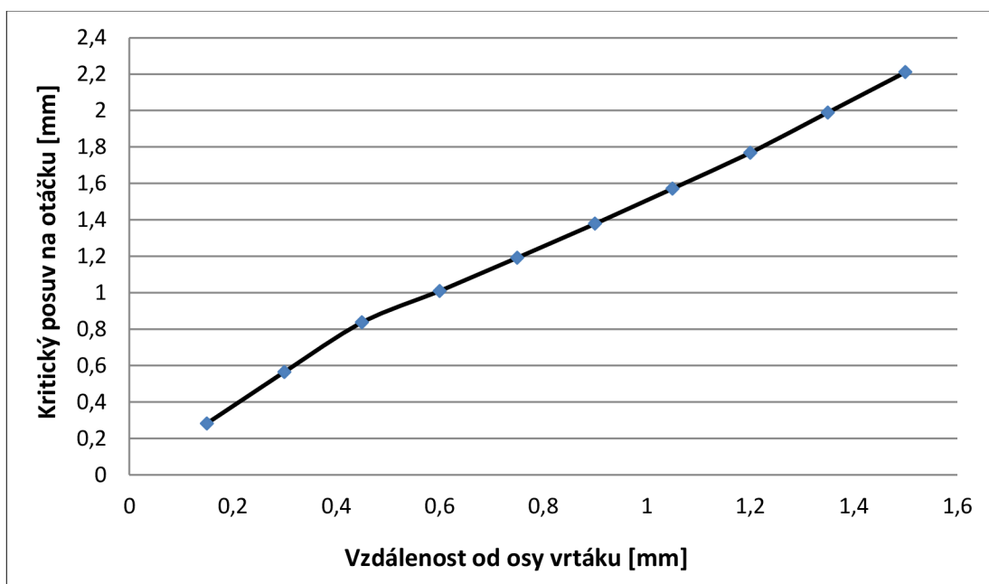
Obr. 4.18 Průběh maximálního posuvu na otáčku podél břitu vrtáku.
