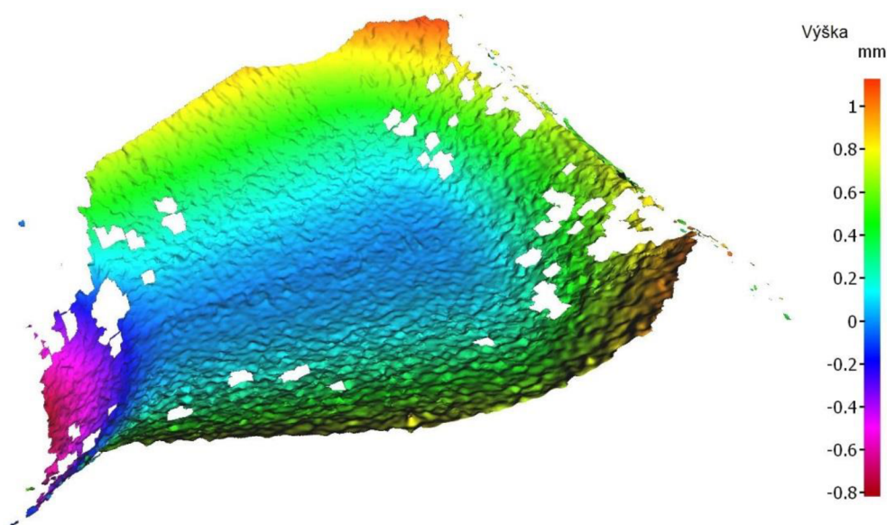
Obr. 4.49 Povrch kuželového přechodu při n = 3500 \text{ min}^{-1} a f = 0,05 \text{ mm} .
