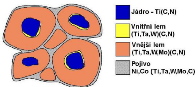
Obr. 3.3 Struktura cernetu [8].
