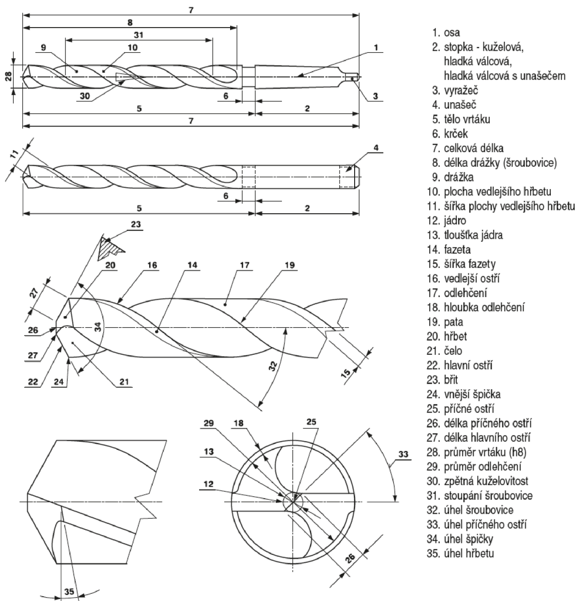
Obr. 1.2 Názvoslovní jednotlivých částí šroubovitého vrtáku [3].
