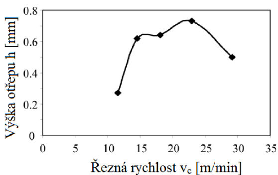
Obr. 1.19 Závislost výšky otřepu na řezné rychlosti [11].
