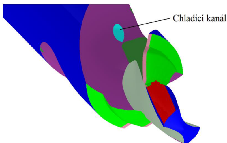
Obr. 4.12 Simulace navrženého stupňovitého vrtáku.
