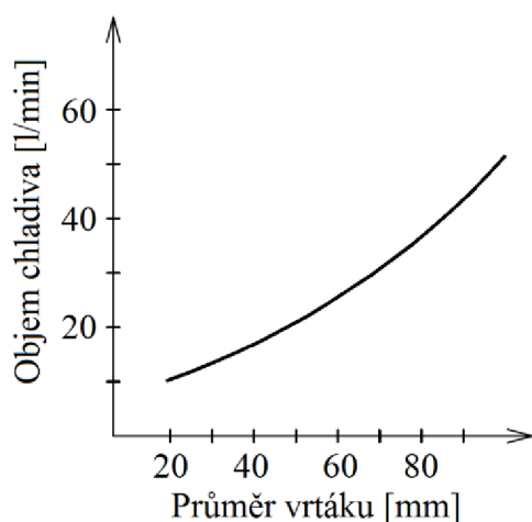
Obr. 1.25 Závislost objemu chladiva na průměru vrtáku [1].
