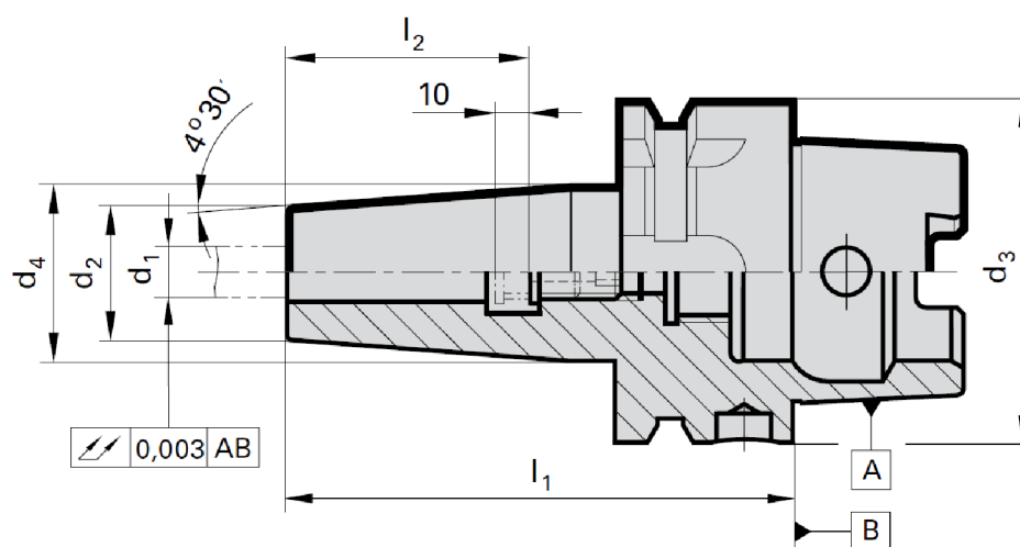
Obr. 4.23 Geometrie upínače HSK-A [31].
