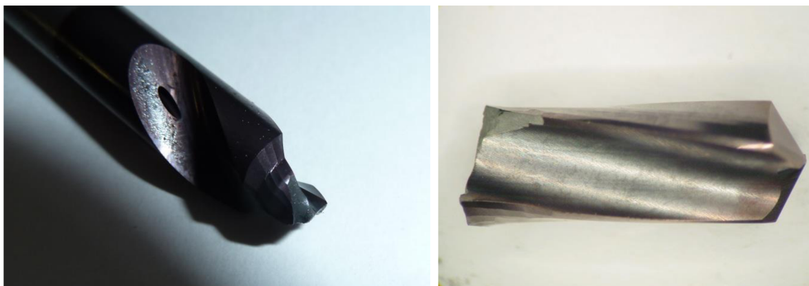
Obr. 4.48 Zlomený vrták.
