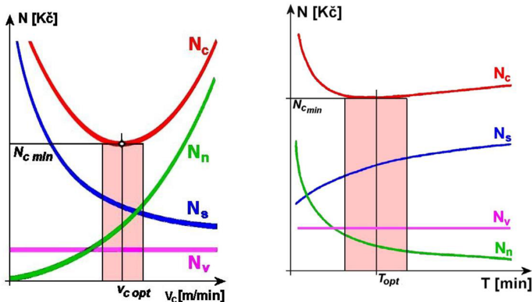
Obr. 2.3 Závislost nákladů na řezné rychlosti [8]. Obr. 2.4 Závislost nákladů na trvanlivosti [8].
