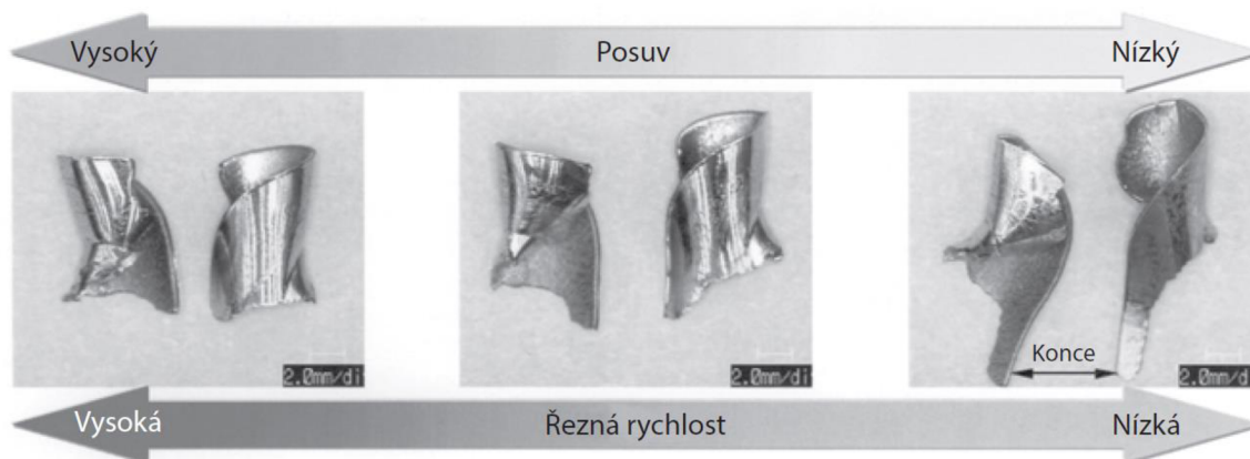
Obr. 1.14 Změna tvaru třísky v závislosti na řezných parametrech [9].
