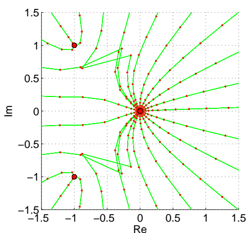
Obrázek 9.1: Lokalizace kořenů polynomu x^5 + 2x^4 + 2x^3 = 0 .
