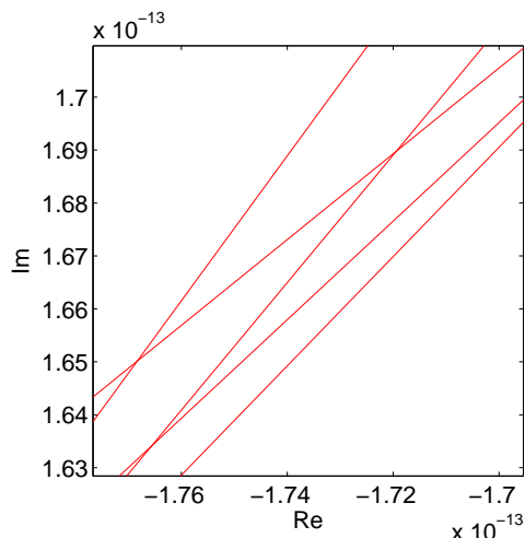
Obrázek 9.4: Detail křivky obrazu dané polynomem (2.1).
