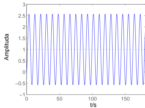
Obrázek 6.8: Přechodová charakteristika systému na mezi stability.
