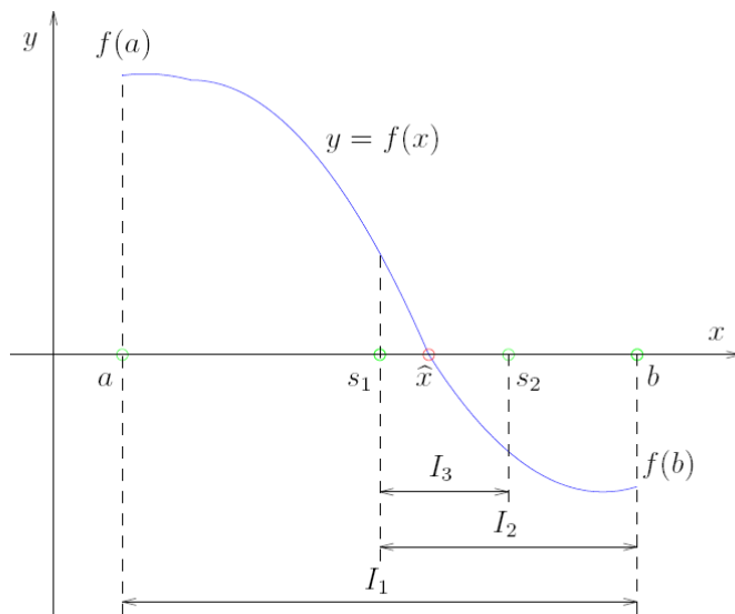
Obrázek 4.2: Princip metody půlení intervalu.
