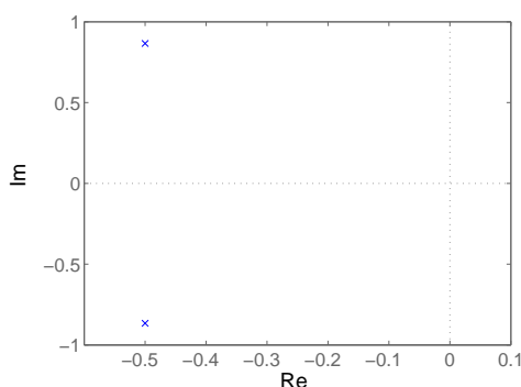
Obrázek 6.6: Rozložení nul a pólů RLC obvodu.
