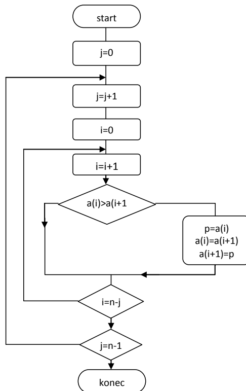
Obrázek 7.4: Vývojový diagram metody Buble sort.
