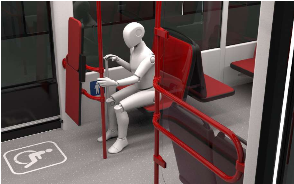
Obr. 6. 26 Madla pro asistenci u sedadel
