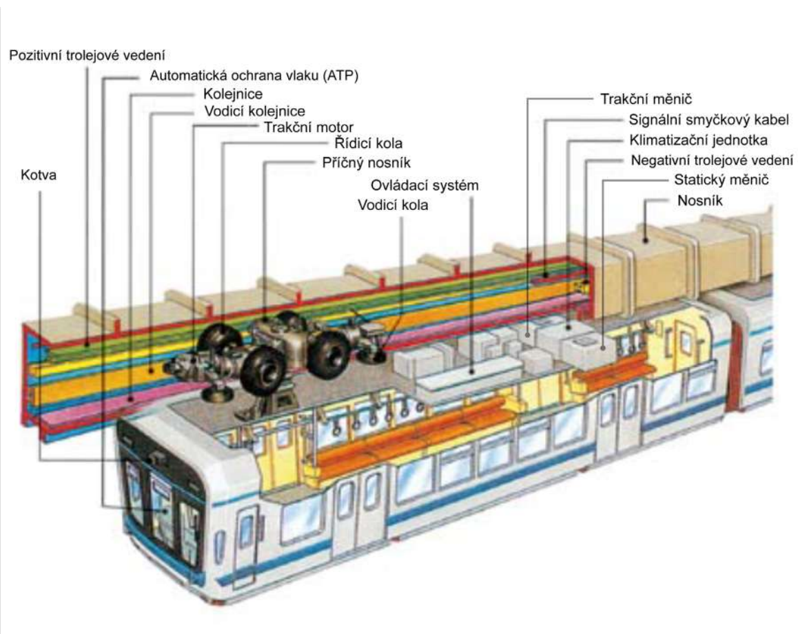
Obr. 2. 28 Schéma SAFEGE systému [40] (upraveno)
