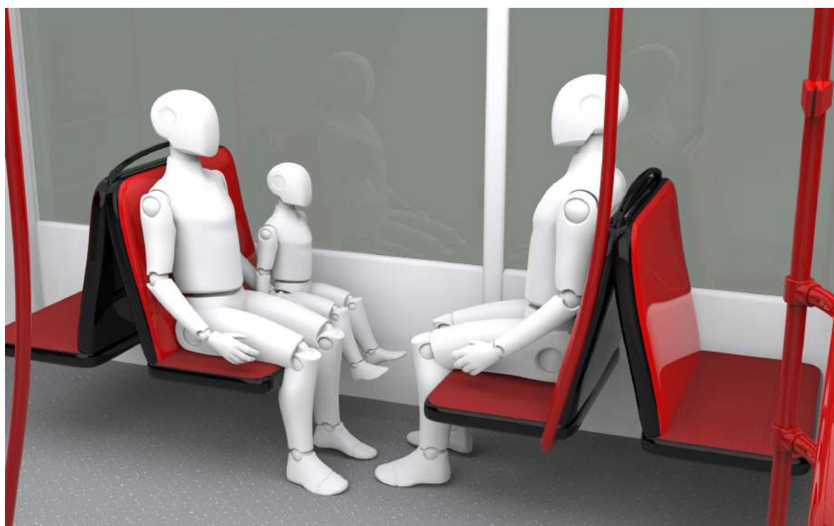
Obr. 6. 18 Perspektivní pohled na čtyřsedadlo
