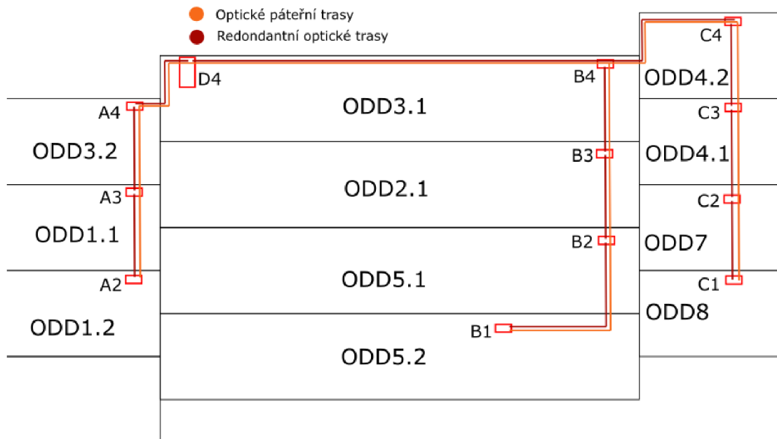
Obrázek č.9 Návrh optických a redundantních tras (Zdroj: vlastní zpracování)
