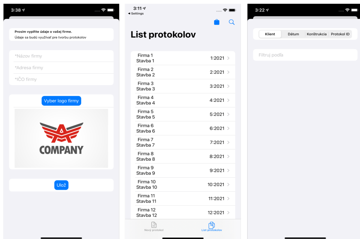
Obr. 5.2: Zobrazenie protokolov
