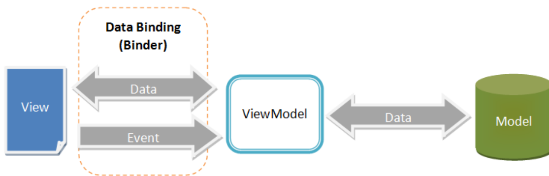
Obr. 3.3: Ukážka komunikácie v rámci MVVM [8]
